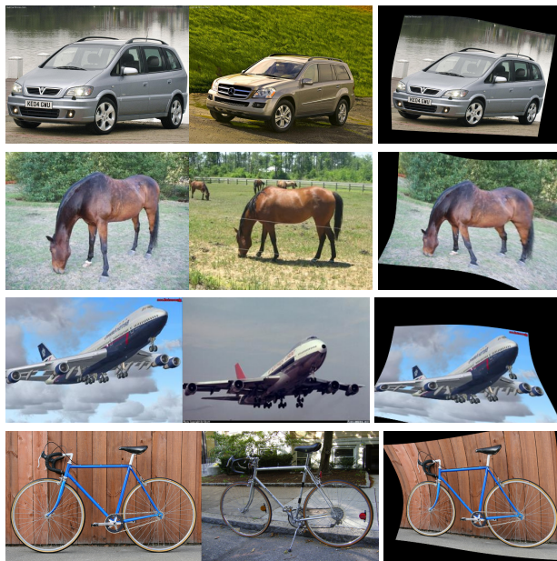
(b) TSS
