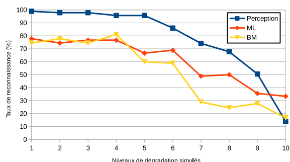
(a) Taux de reconnaissance du mot en première position
