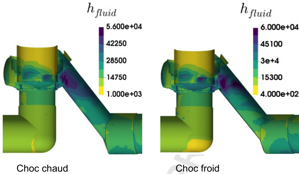
Fig. 2. Champs de coefficient d'échange thermique ( W/m^2K ).
