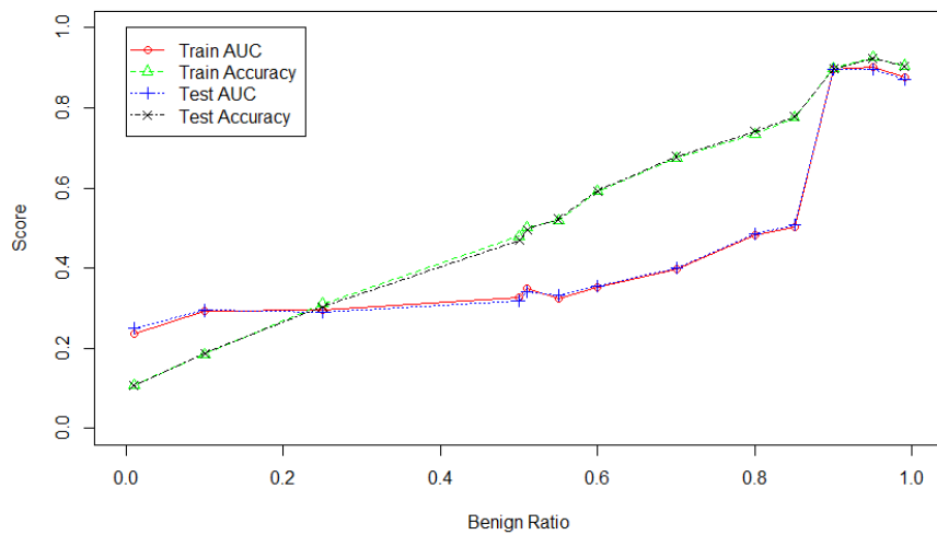
Fig. 5: MCD
