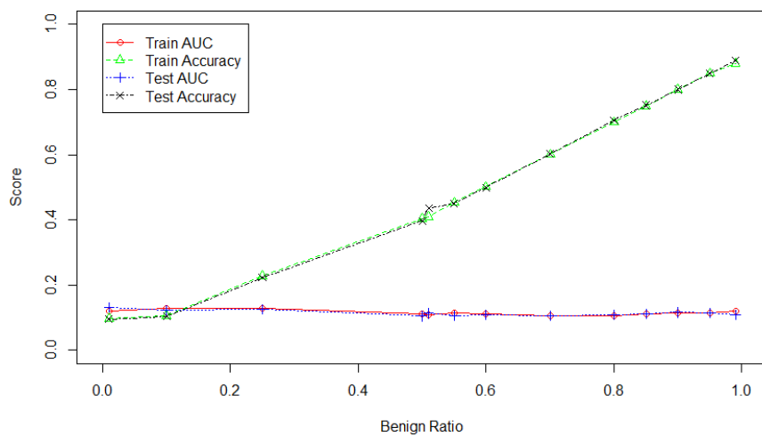
Fig. 6: OCSVM
