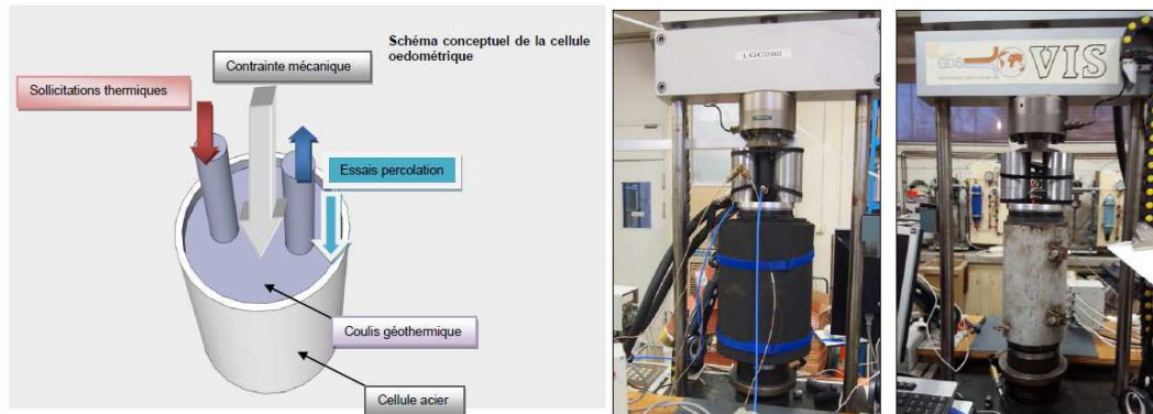
Figure 1. Schéma conceptuel et développement de la cellule œdométrique.
