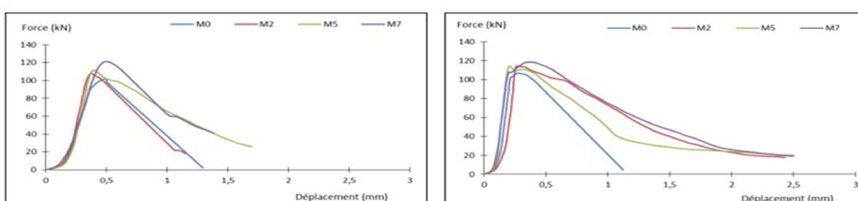
Courbes force-déplacement en compression (éprouvettes non pré-fissurées).
