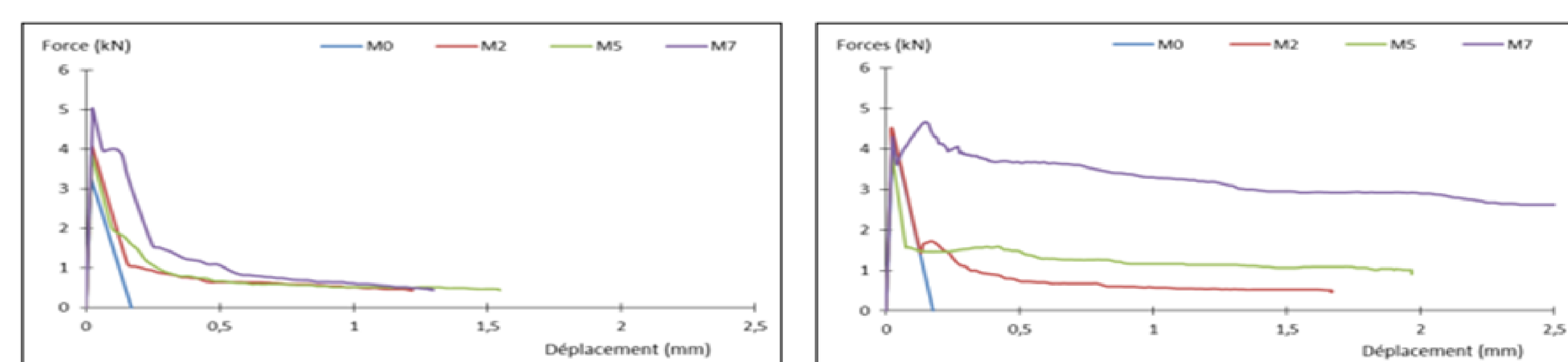
Courbes force-déplacement en flexion (éprouvettes non pré-fissurées).
