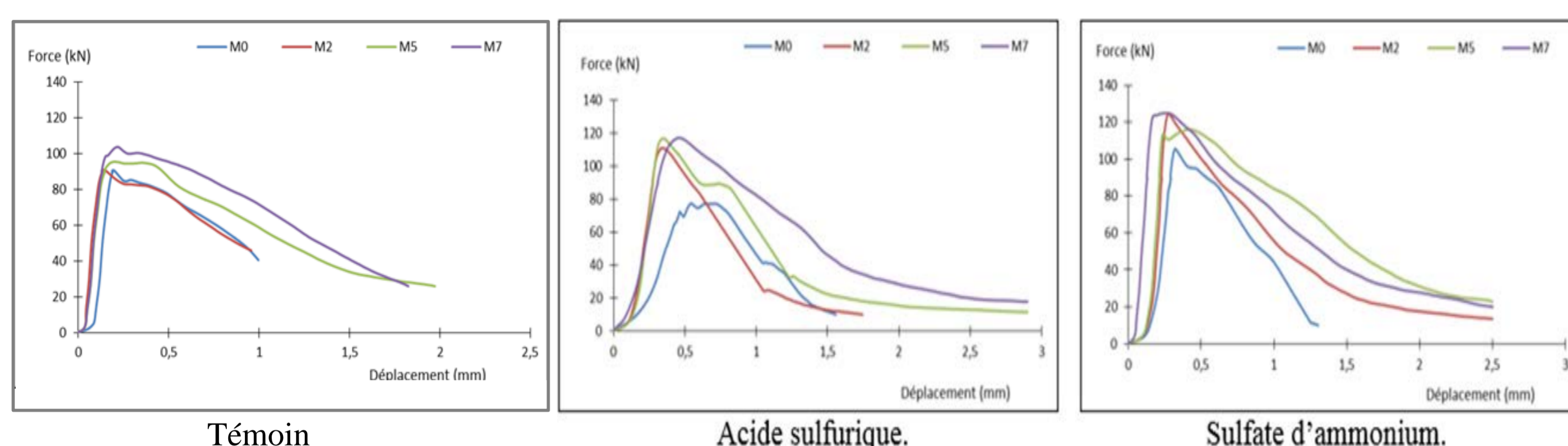
Courbes force-déplacement en compression (éprouvettes non pré-fissurées).
