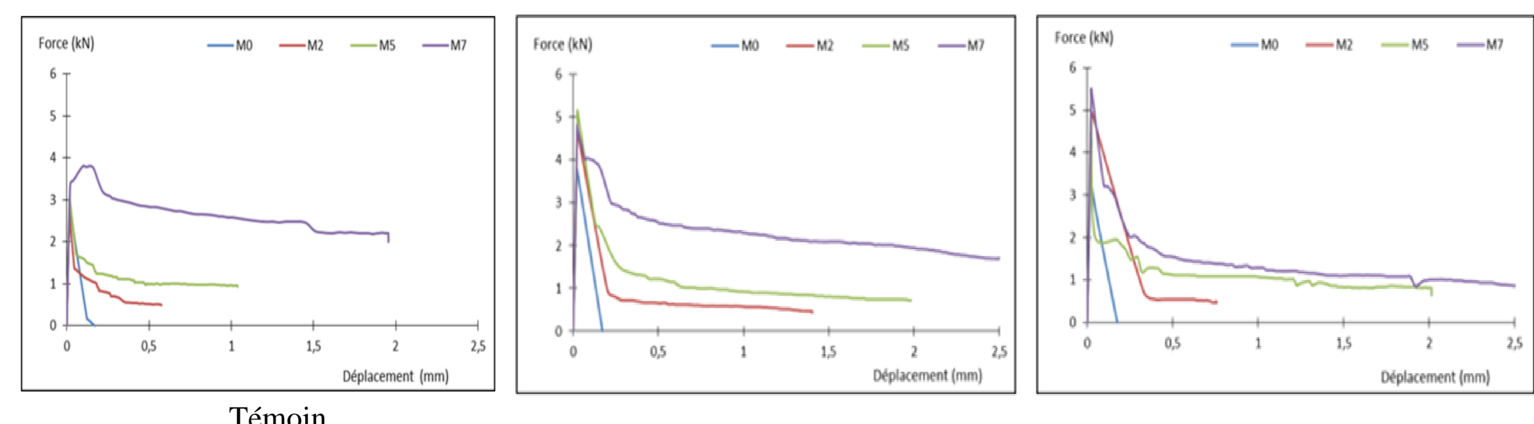
Courbes force-déplacement en flexion (éprouvettes non pré-fissurées).
