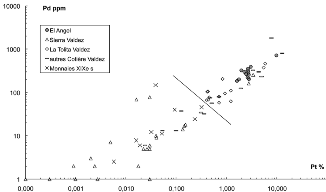
Figure 4 : Représentation des concentrations en Pd et en Pt (en ppm) pour la figurine d'El Angel et pour divers objets de La Tolita Tumaco et d'Esmeraldas publiés par Barrandon et al. , 2004 et par Valdez et al. , 2005 et des monnaies sud américaines (Guerra, 2004b).
