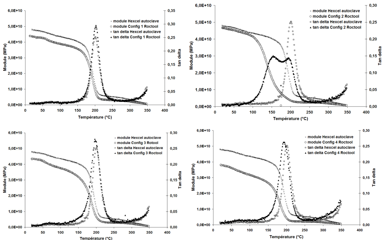
Fig. 8. Comparaison par DMA de plaques fabriquées par autoclave et par le procédé Roctool selon différents cycles de cuisson.
