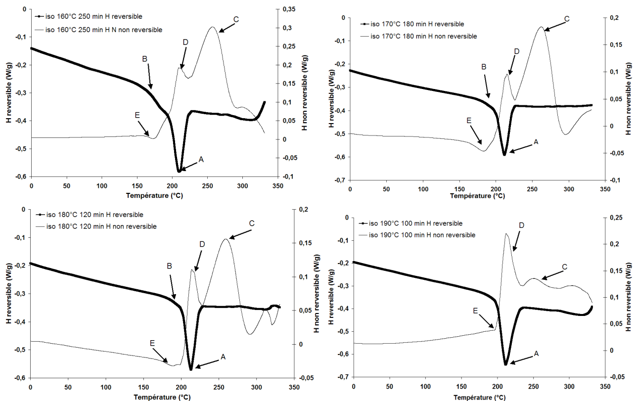
Fig. 3. Balayage résiduel MDSC à 10 °C/min de résine M21 après cuisson isotherme à 160, 170, 180 et 190 °C. Fig. 3. Residual modulated DSC scan at 10 °C/min of M21 resin samples after isothermal curing at 160, 170, 180 and 190 °C.
