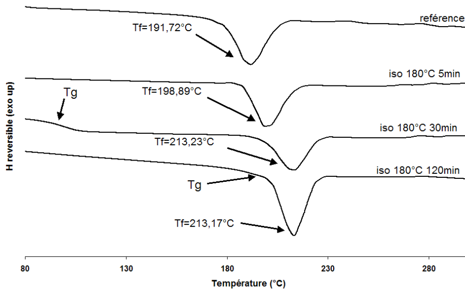
Fig. 5. Évolution de la température de fusion en fonction du temps de cuisson.
