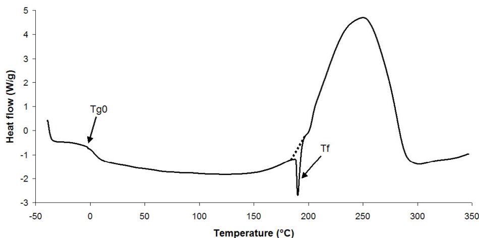
Fig. 1. Balayage DSC 10 °C/min de la résine M21 non renforcée.
