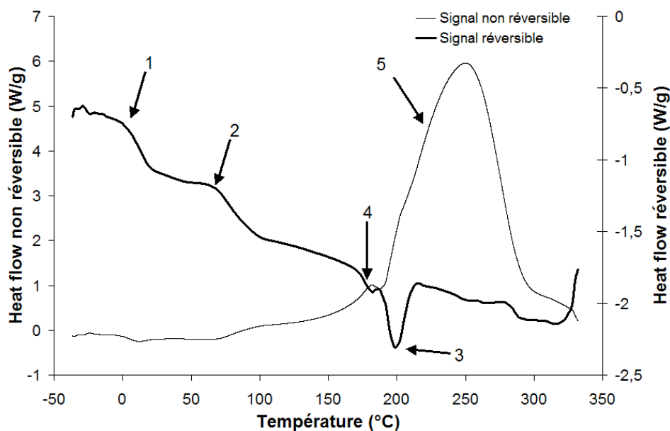
Fig. 2. Thermogramme de la résine M21 obtenu par DSC modulée à 10 °C/min.
