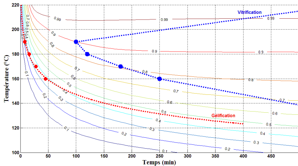
Fig. 6. Diagramme TTT isotherme de la résine M21 non renforcée.
