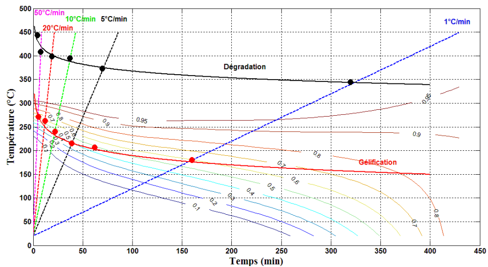
Fig. 7. Diagramme TTT dynamique de la résine M21.
