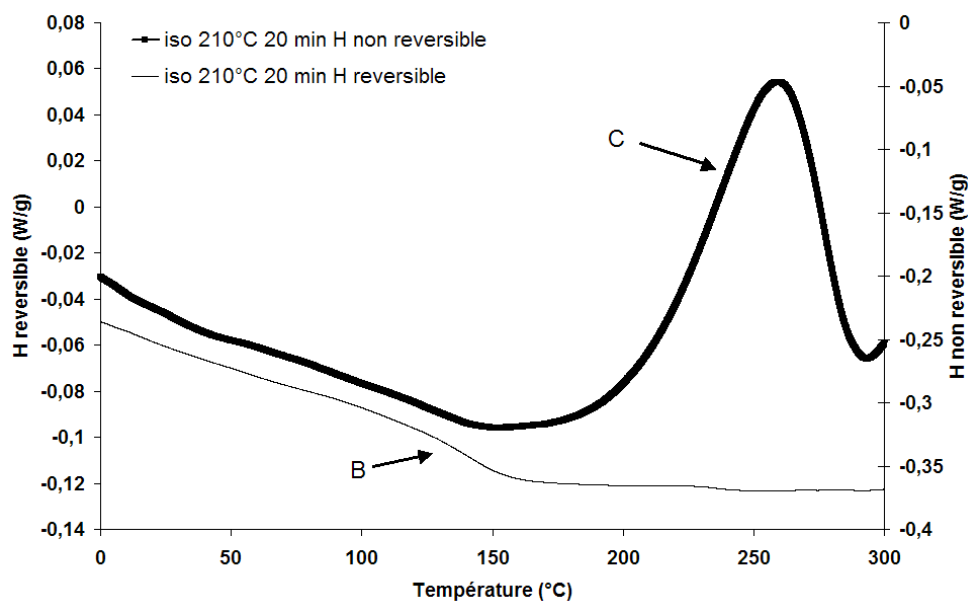
Fig. 4. Balayage résiduel MDSC à 10 °C/min après cuisson isotherme à 210 °C.
