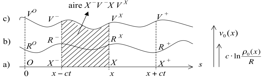
FIGURE 5 – Représentation géométrique arbitraire de l'état de l'air à partir des conditions initiales : a) tuyau ; b) échelle des densités ; c) échelle des vitesses.
