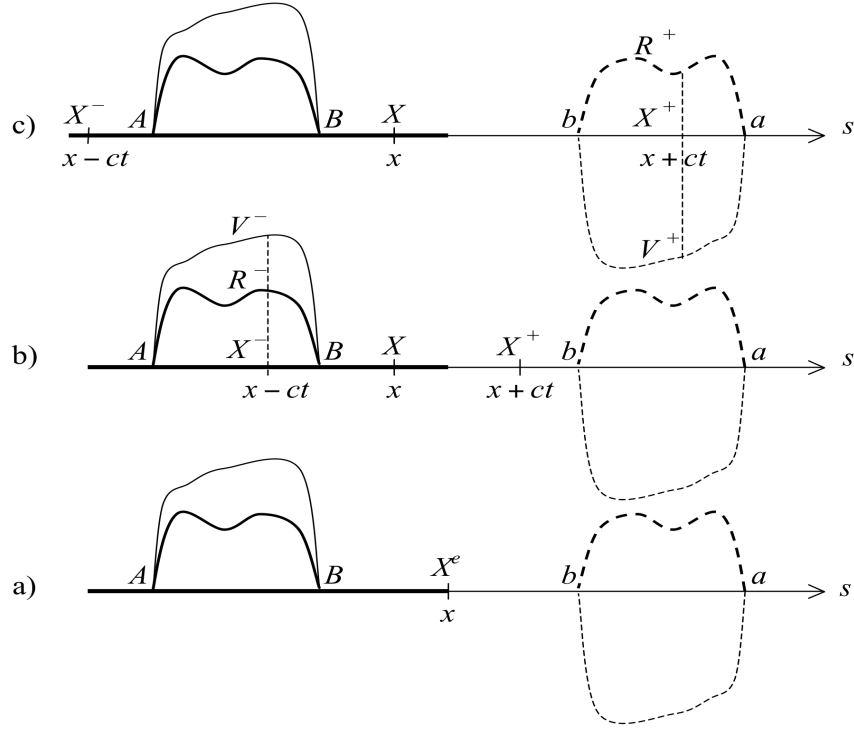
FIGURE 6 – Propagation d’un son dans un tuyau fermé à son extrémité droite (en gras, échelle des densités) : a) perturbations initiales réelles (lignes continues) et imaginaires (lignes discontinues) ( t = 0^+ ); b) perception à la position x du premier son ( \frac{BX}{c} \leq t \leq \frac{AX}{c} ); c) perception à la position x du deuxième son ( \frac{Xb}{c} < t < \frac{Xa}{c} ) : l’écho.
