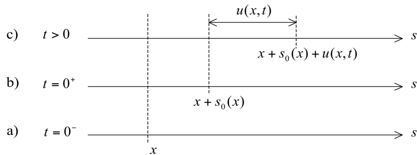
FIGURE 3 – Position d'une particule d'air dans le tuyau : a) au repos ; b) initialement, quand l'équilibre de l'air est perturbé ; c) après perturbation initiale.
