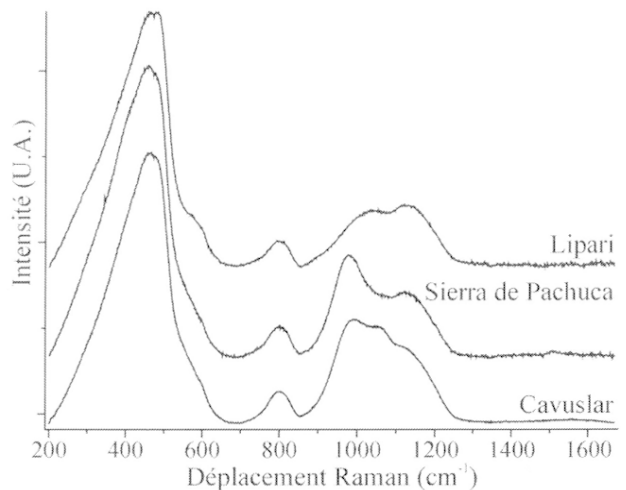
Fig. 7 : Spectres Raman des  chantillons Cavuslar, Sierra de Pachuca et Lipari de la figure 6 apr s le retrait des lignes de bases destin es   s'affranchir des fonds continus.
