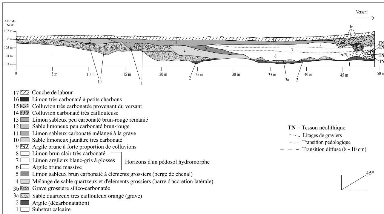
Fig. 6. Coupe du chenal sud (tranche 2). D'après DAGOBERT et alii, 2001.
