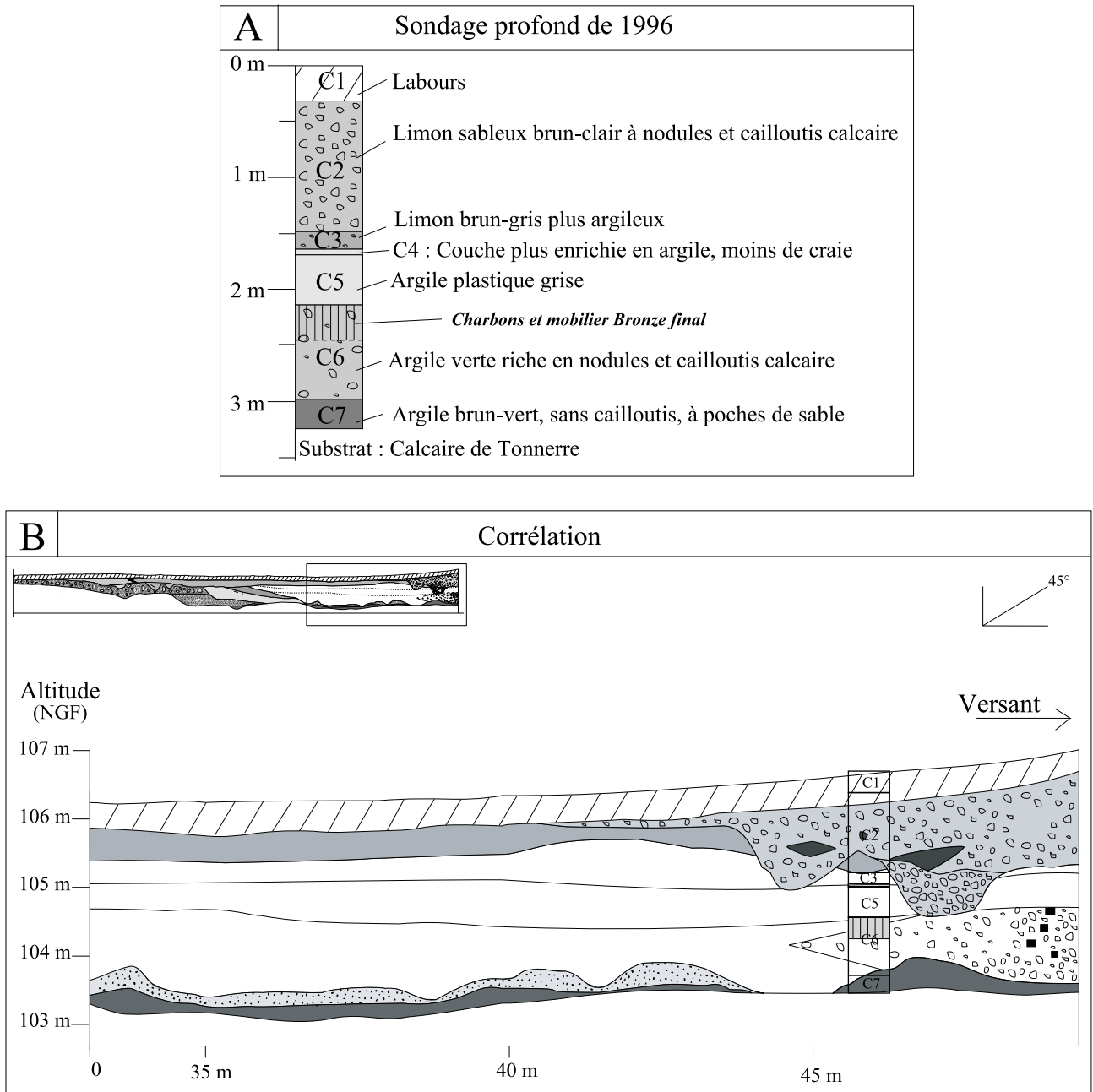
Fig. 8. Corrélation entre le sondage profond de 1996 et la coupe de la tranchée 2 (chenal sud). A. d'après DUHAMEL, 1996 ; B. d'après DAGOBERTE et alii, 2001.
