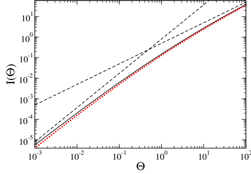
FIGURE 3: Dans l'approximation de taux (53), loi d'interpolation (trait plein) raccordant le régime superdiffusif ( \Theta \ll 1 ) et le régime diffusif ( \Theta \gg 1 ) de l'étalement sous-balistique de la phase du condensat à très faible \nu ( \nu \rightarrow 0^- à \Theta fixé) sous l'effet des collisions Landau-Khalatnikov aux petits angles. Le temps renormalisé \Theta est celui de l'équation (70), et la fonction représentée est l'intégrale I(\Theta) au second membre de l'équation (71). En tireté : comportements aux limites I(\Theta) \sim \frac{3}{10}\Gamma(1/3)\Theta^{5/3} pour \Theta \rightarrow 0 et I(\Theta) \sim \frac{1}{2}\Theta pour \Theta \rightarrow +\infty . Disques rouges : résultats numériques pour \nu = -1/10 tirés de l'expression exacte (78) et soumis au même redimensionnement que dans l'équation (71) (on donne C(\nu = -1/10) = 2,596\,303\dots et X(\nu = -1/10) = -75,909\,694\dots ).
