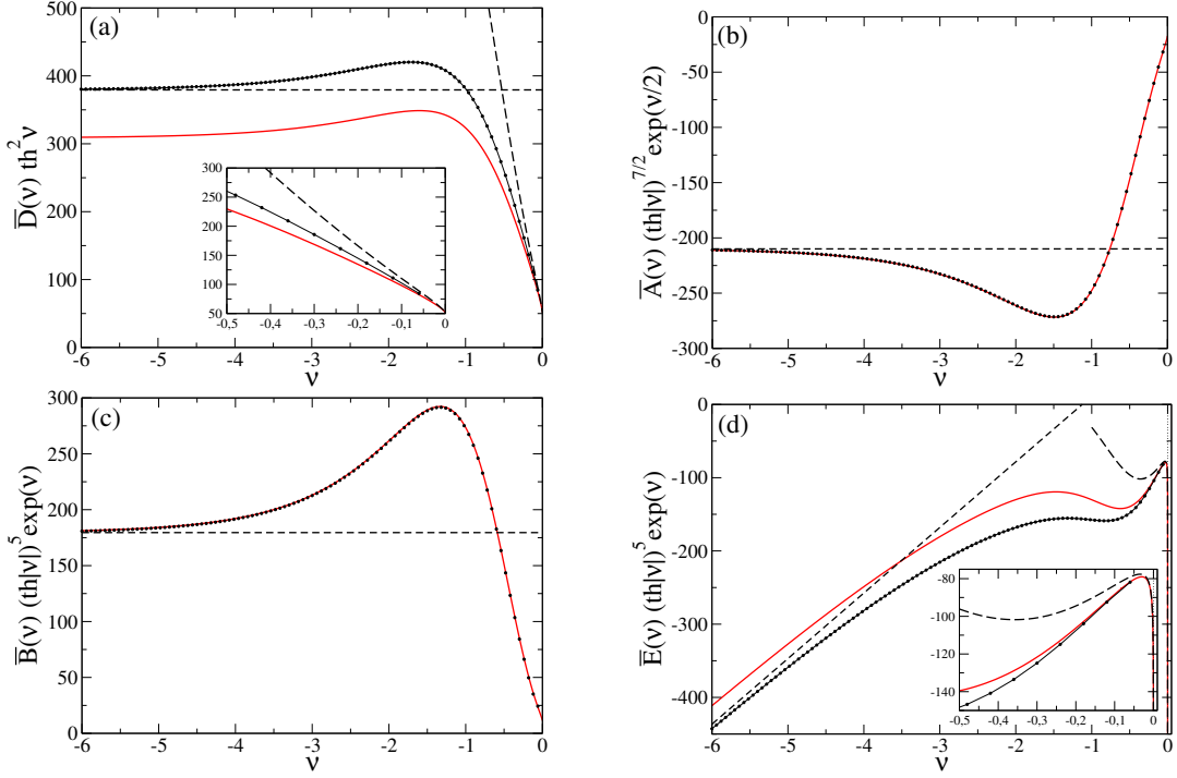
FIGURE 2: Coefficients \bar{D} , \bar{A} , \bar{B} et \bar{E} du développement aux temps longs de la variance sous-balistique du déphasage du condensat, voir les équations (72) et (57), en fonction du potentiel chimique réduit \nu = \mu_\phi/k_B T du gaz de phonons. Ici la branche acoustique a un départ concave et les processus collisionnels entre phonons pris en compte sont ceux de Landau-Khalatnikov aux petits angles. Disques noirs (avec parfois une fine ligne directrice) : résultats exacts obtenus numériquement. Trait plein rouge : résultats (58,59,60,61) dans l'approximation de taux. Tireté : comportements aux limites (89,90) et (96,97,98,99) prédits analytiquement. Les coefficients sont multipliés par les puissances de \text{th}|\nu| et de e^\nu leur conférant des limites finies et non nulles en \nu = 0 et \nu = -\infty . Les vignettes sont des agrandissements.
