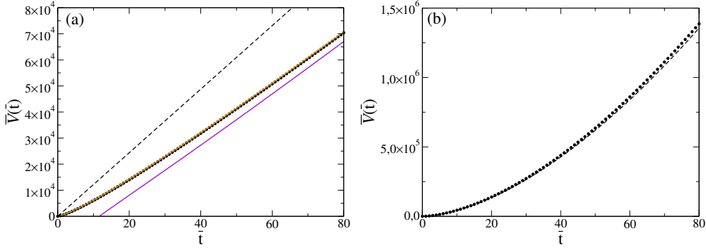
FIGURE 4: Variance réduite sous-balistique \bar{V}(\bar{t}) du déphasage du condensat en fonction du temps, obtenue par diagonalisation numérique de \hat{\mathcal{H}} dans l'équation (52), pour un potentiel chimique des phonons réduit (a) \nu = -1/2 , (b) \nu = 0 . Disques noirs : résultats numériques. Tireté : (a) partie diffusive exacte \bar{D}\bar{t} ; (b) : équivalent asymptotique d_0^{\text{app}}\bar{t}^{5/3} prédit par l'approximation de taux, voir les équations (64,65). Trait plein violet dans (a) d'aspect rectiligne : développement asymptotique (72) exact à o(1) près. Trait plein orange dans (a) : approximation hybride de \bar{V}(\bar{t}) , somme de la partie diffusive numérique \bar{D}\bar{t} et de la partie sous-diffusive dans l'approximation de taux.
