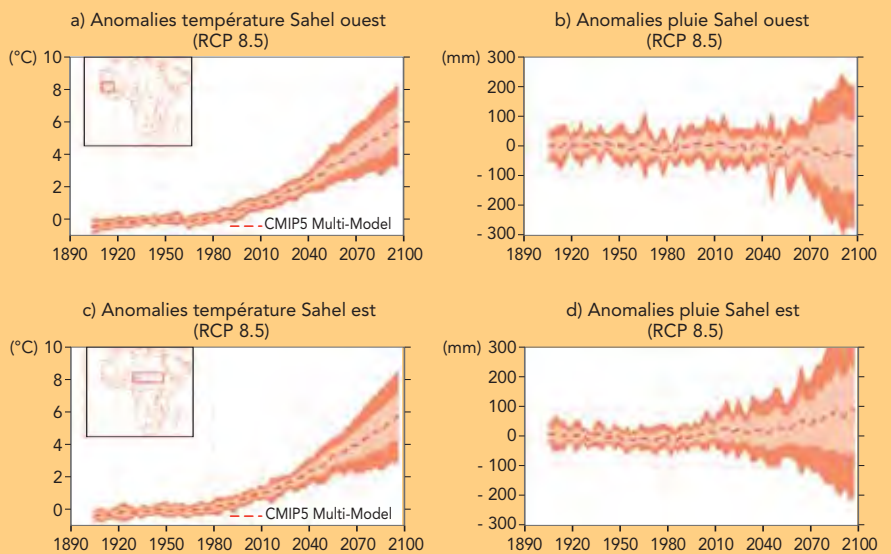
Figure 16. Les projections climatiques de température et de précipitations au Sahel ouest et est, pour le scénario RCP 8.5. L'évolution projetée de la température est nettement positive pour l'ensemble des modèles, alors que les projections de précipitations sont très incertaines.
