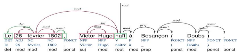
En rouge le chemin le plus court, en vert les tokens récupérés sur le chemin.
