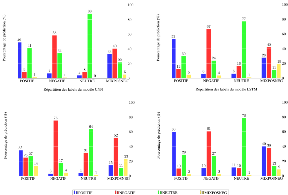
FIGURE 2 – Répartition des prédictions par label de référence des différents modèles de la tâche 2
