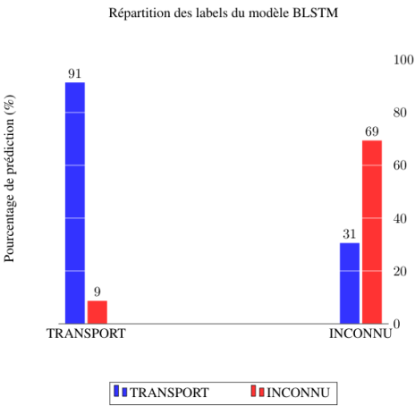
FIGURE 1 – Répartition des prédictions par label de référence du modèle BLSTM de la tâche 1
