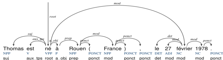
FIGURE 5 : Exemple de phrase sélectionnée après analyse syntaxique
