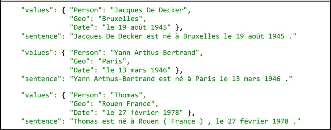
FIGURE 8 : exemples de valeurs trouvées par le patron “.* est né à .* le .*”
