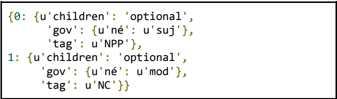
FIGURE 4 : Exemple de patron syntaxique correspondant au patron lexical “.*, né le .*” Chaque entrée du patron correspond à une entité à extraire et ses attributs attendus
