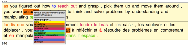
FIGURE 3: Interface de l'outil Yawat permettant d'effectuer l'annotation.
