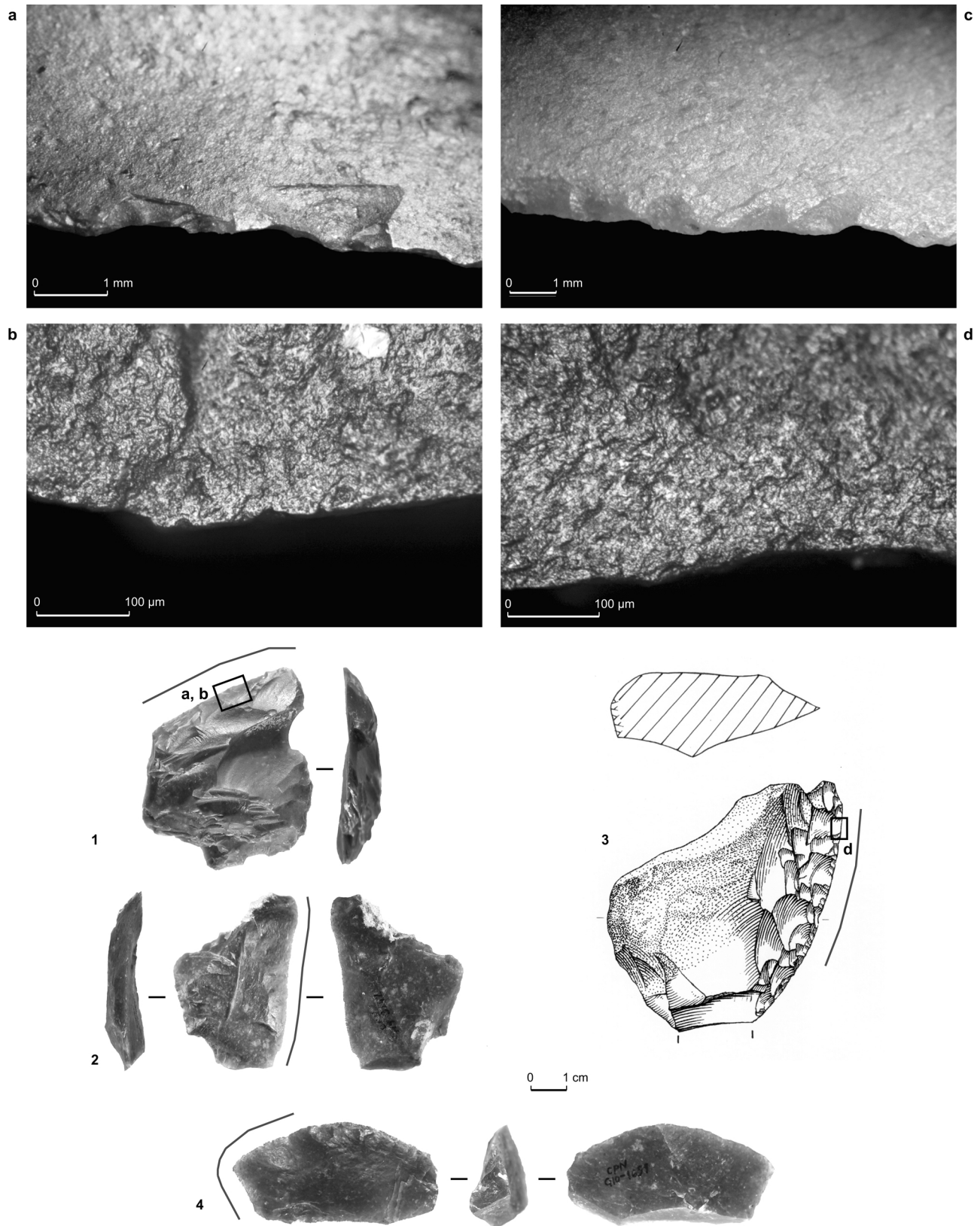
Fig. 5 – Pièces ayant servi à couper des matières tendres à mi-dures carnées et traces d'utilisation associées. a et c, esquillements ; b et d, micro-polis. 1, racloir sur éclat en Turonien détaché par percussion marginale ; 2, éclat brut en Sénonien brun ; 3 et 4, racloirs Quina en Sénonien brun (dessin : S. Pasty).
