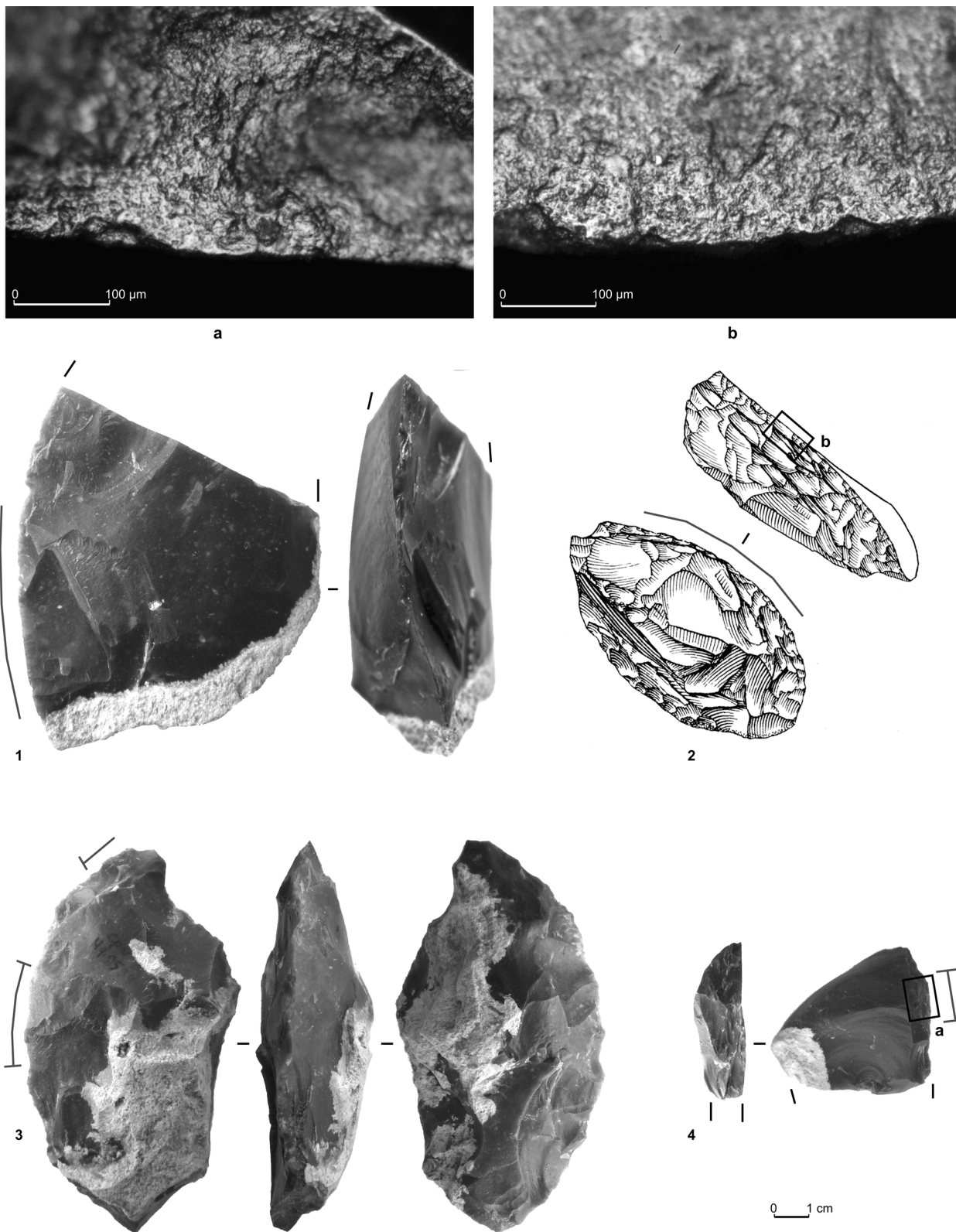
Fig. 2 – Raclours ayant servi à la découpe de matières tendres cutanées, et exemples de poliss de découpe cutanée. 1, raclour Quina sur éclat débité par percussion interne volontairement fracturé ; 2, raclour Quina sur éclat débité par percussion interne ; 3, raclour sur support bifacial ; 4, fragment de raclour repris depuis sa partie proximale par un enlèvement outrepassant et dont le tranchant a été ravivé. 1, Sénonien brun ; 2 à 4, Sénonien noir (dessin : S. Pasty). Scrapers used for skin cutting, and corresponding use-wear traces. 1, Quina scraper intentionally fractured and made out of a flake with internal percussion; 2, Quina scraper made out of a flake with internal percussion; 3, bifacial scraper; 4, scraper fragment modified from the proximal part by a bypassing removal and with a resharpened edge. 1, brown Senonian flint; 2 to 4, Black Senonian flint (drawings: S. Pasty).
