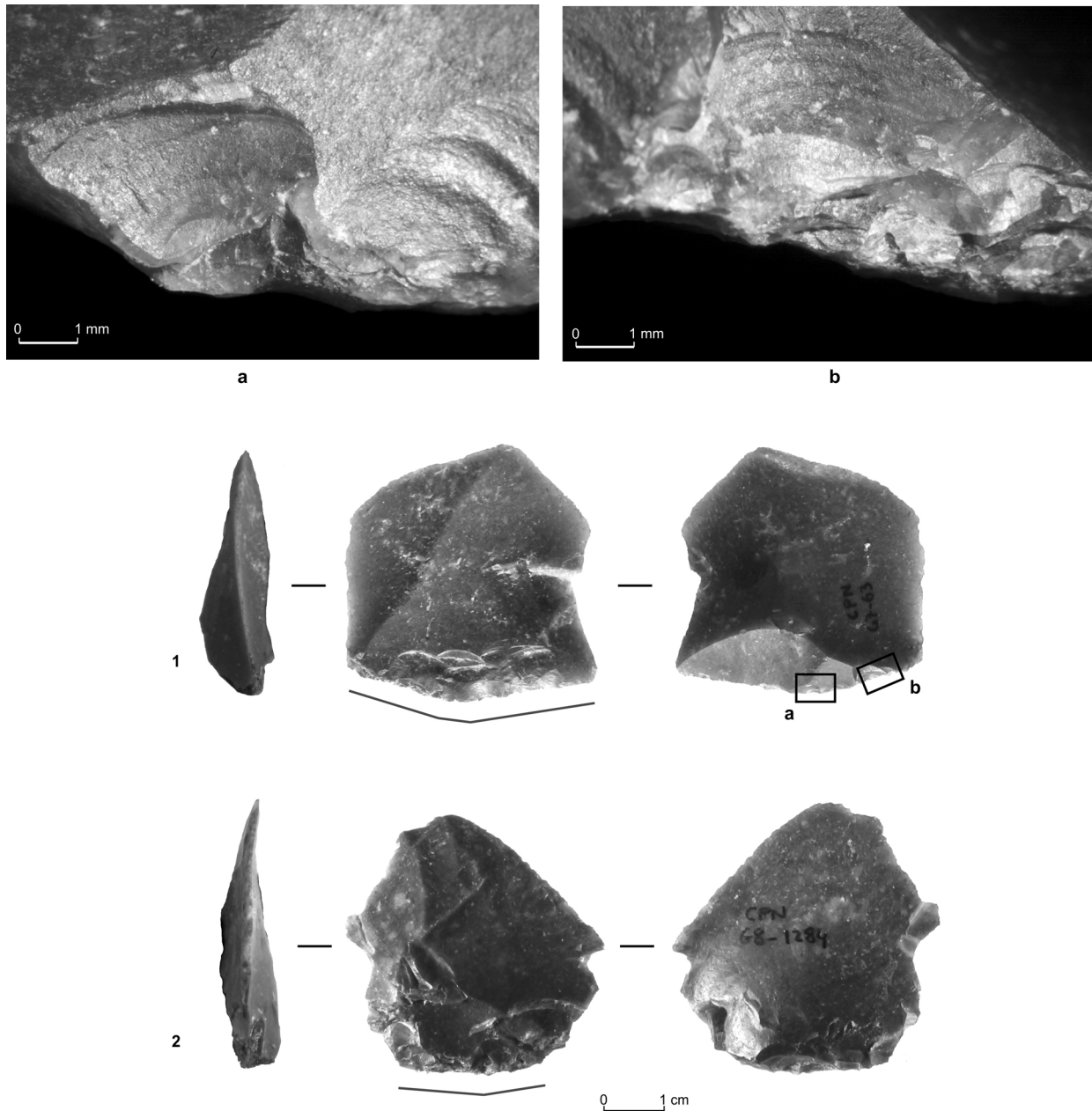
Fig. 10 – Éclats de dénaturation présentant des traces de percussion contre des matières dures mixtes (organiques et minérales) sur le tranchant de l'ancien racloir. a, esquillements ; b, esquillements et écrasements ; 1, Sémonien brun ; 2, Sémonien noir.
