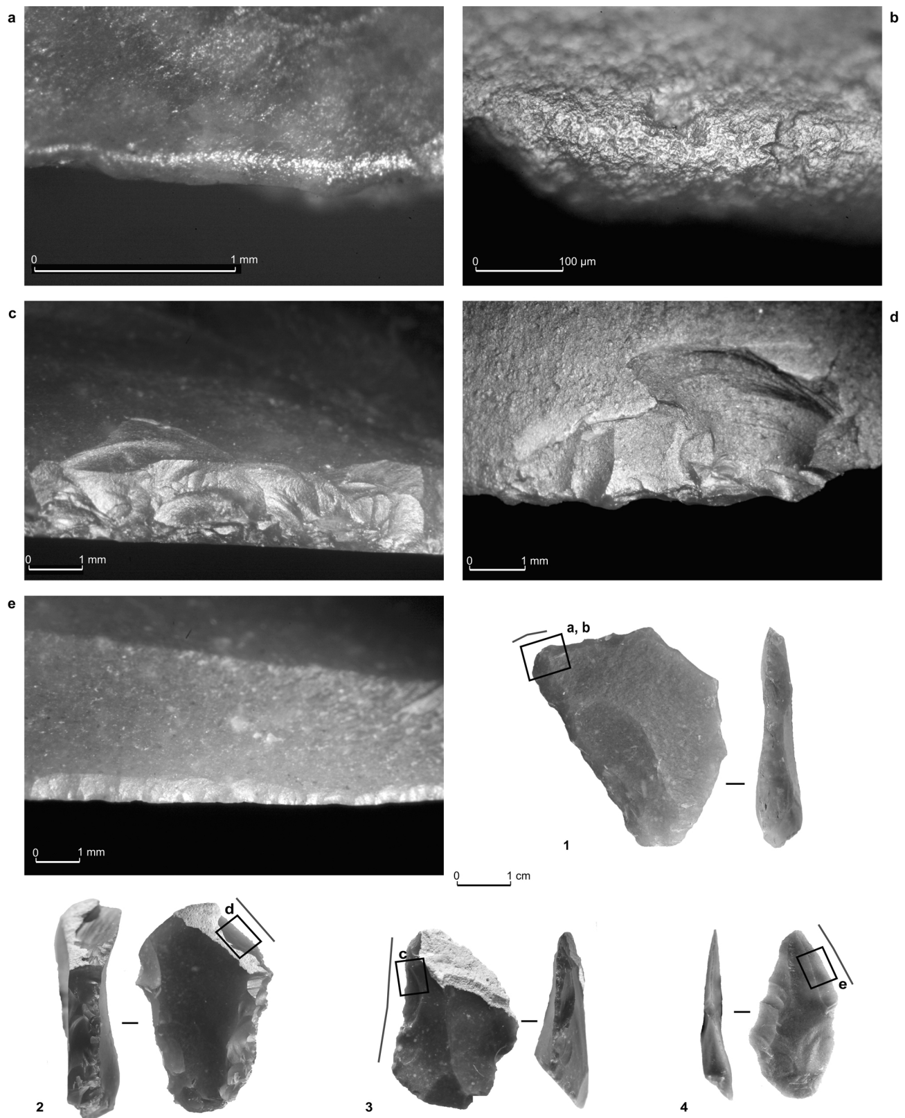
Fig. 8 – Pièces utilisées pour effectuer des actions transversales et traces d'utilisation associées. a, macro-émoussé ; b, micro-émoussé et poli ; c, d, et e, esquillements ; 1, racloir sur éclat probablement détaché par percussion marginale en Sénonien brun, utilisé pour racler de la peau sèche ; 2, racloir sur éclat détaché par percussion interne en Turonien, utilisé sur un bord brut pour racler une matière dure organique en coupe positive ; 3, probable éclat de dénaturation en silex Sénonien noir utilisé pour racler une matière dure organique en coupe négative ; 4, éclat détaché par percussion marginale ayant servi à racler une matière tendre à mi-dure en coupe négative.
