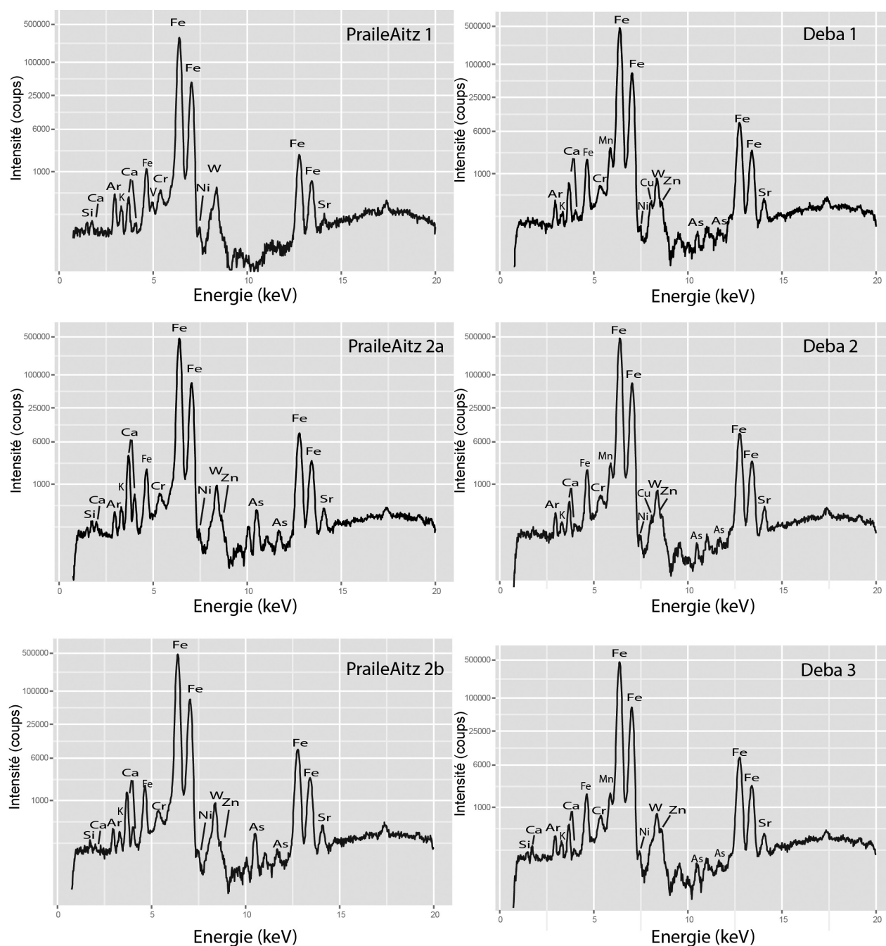
Fig. 5. Spectres XRF des trois blocs facettés de Praileaitz I et de trois galets d'ocre collectés le long du Deba. Le pic de tungstène (W) est produit par l'anticathode du tube X de l'appareil. Les pics de fer (Fe) proches du strontium (Sr) et du chrome (Cr) sont des artefacts liés à la très grande teneur en fer des échantillons. Ils masquent certains autres éléments. / XRF spectra obtained on the three modified ochre lumps from Praileaitz I and three ochre lumps collected on the Deba riverbank. The peak of tungstene (W) is produced by the anticathode of the X-ray tube. Iron peaks (Fe) close to strontium (Sr) and chromium (Cr) are due to the high concentration of iron and mask some other elements.
