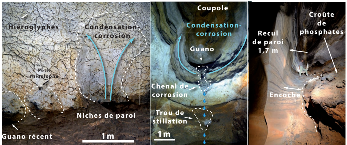
Figure 15 : Niches de paroi et encoches formées par les convections d'air produisant de la condensation-corrosion en présence de chauves-souris. À gauche : niches en pied de paroi au-dessus de guano ancien et frais, un petit rhinolophe est visible en haut de la niche centrale, grotte de Saint-Marcel, Ardèche. Cliché Cailhol. Au centre : sous une grande coupole de plafond, du guano est accumulé à la base de la niche. Les percolations de condensation produites au sommet de la coupole se collectent dans un chenal de corrosion après avoir traversé le guano acide. Les percolations du chenal s'égouttent ensuite et forment un trou de stillation, grotte de Saint-Marcel, Ardèche. Cliché D. Cailhol.
