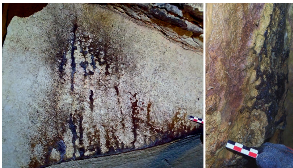
Figure 5 : Altération des parois liée aux excréments de chauves-souris. Échelle à graduation centimétrique. À gauche : cupules et rigoles s'approfondissant vers le bas, grotte d'Azé, Saône-et-Loire. À droite : profondeur d'altération des parois liée aux excréments de chauves-souris, grottes de Blanot, Saône-et-Loire. Cliché L. Barriquand. Weathering of walls made by bats excrements. Scale with centimetric graduation. Left: cupules and rills going deeper downwards, grotte d'Azé, France. Right: weathering depth of the walls made by bat excrements, grottes de Blanot, France.
