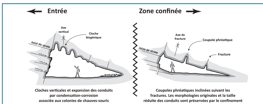
Figure 27 : Types de coupoles, avant le bouchon de calcite et confinées derrière, grotte d'Azé, Saône-et-Loire. À gauche : coupoles de la partie ouverte, proche de l'entrée (avant le bouchon), d'origine biologique (chauves-souris) et creusées selon un axe vertical. La galerie s'est de plus agrandie par expansion sous l'effet de la condensation-corrosion. À droite : coupoles de la partie profonde (au-delà du bouchon), d'origine phréatique et creusées sur la fracturation. Le conduit est resté dans les dimensions originelles, non influencées par la phase d'expansion tardive liée à la condensation-corrosion. Types of cupolas, outward of the calcite plug and inward in the confined zone, grotte d'Azé, France. Left: cupolas in the outward zone close to the entrance (before the calcite plug); the cupolas are of biologic (bats) origin and develop according to a vertical axis. Moreover, the passage size increased by expansion resulting from condensation-corrosion. Right: cupolas in the inward (confined) zone, beyond the calcite plug; the cupolas are of phreatic origin and develop according to joints, which are inclined. The passage remained in its original size, with no influence of the late phase of expansion through condensation-corrosion that occurred close to the entrance.
