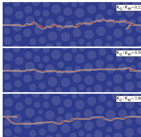
FIGURE 1 – Chemin de fissure dans un échantillon de densité de grain 0.5. Ratio de ténacités grains/matrice (de haut en bas) : 0.25, 0.5, 2.0.
