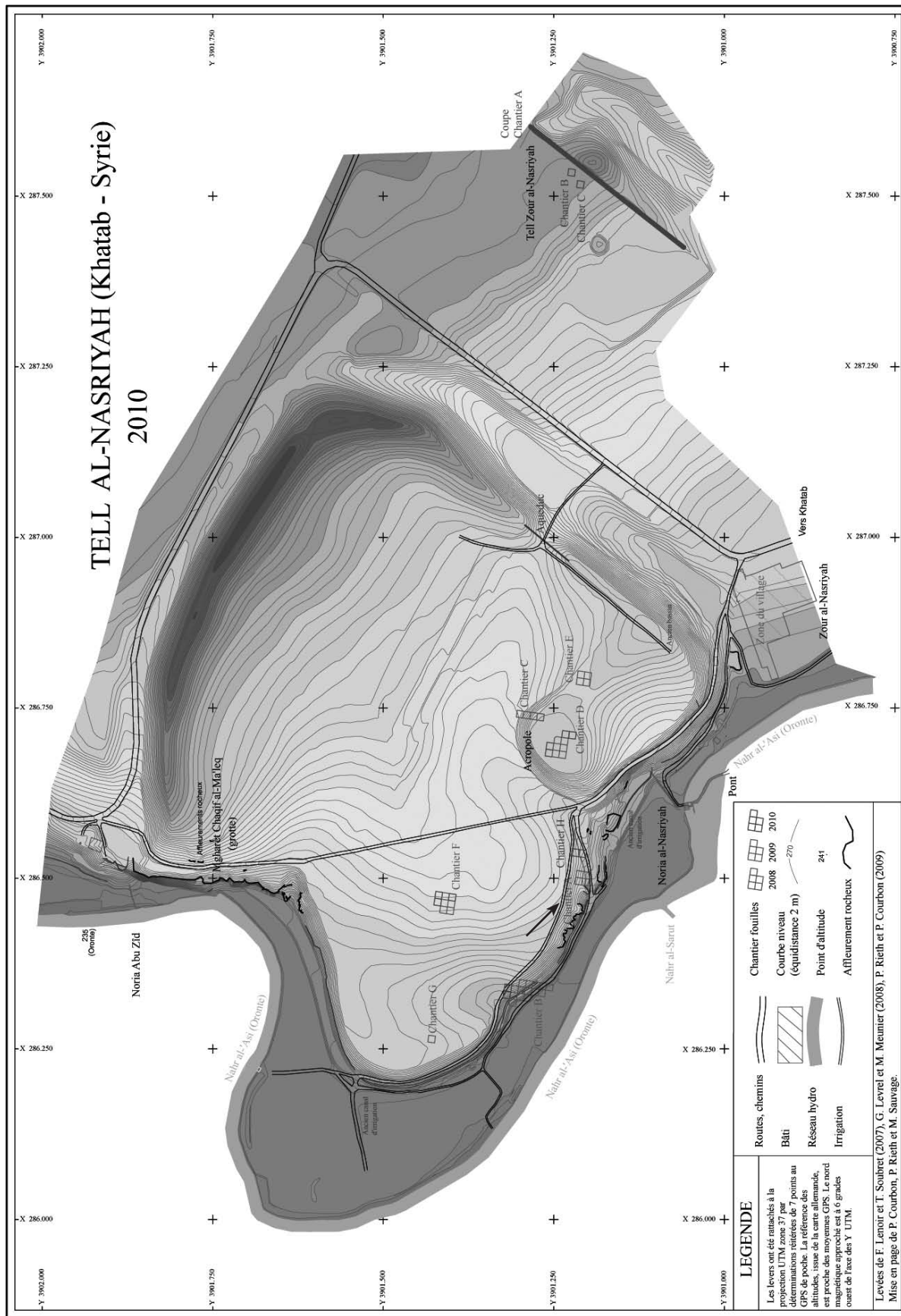
Planche 2.1. Tell al-Nasriyah, relevé topographique : implantation du chantier A (1), © P. Courbon, P. Rieth et M. Sauvage
