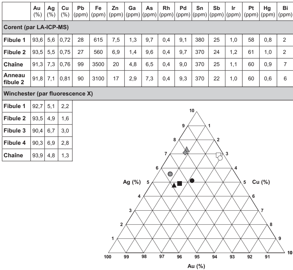
Fig. 7 – Composition métallique des fibules de Corent (méthode LA-ICP-MS) et des fibules du trésor de Winchester (méthode fluorescence X) : représentation en diagramme ternaire et tableau de composition : Au, or ; Ag, argent ; Cu, cuivre ; Pb, plomb ; Fe, fer ; Zn, zinc ; Ga, gallium ; As, arsenic ; Rh, rhodium ; Pd, palladium ; Sn, étain ; Sb, antimoine ; Ir, iridium ; Pt, platine ; Hg, mercure ; Bi, bismuth (tableau et graphique : B. Gratuze et S. Nieto, CNRS).
