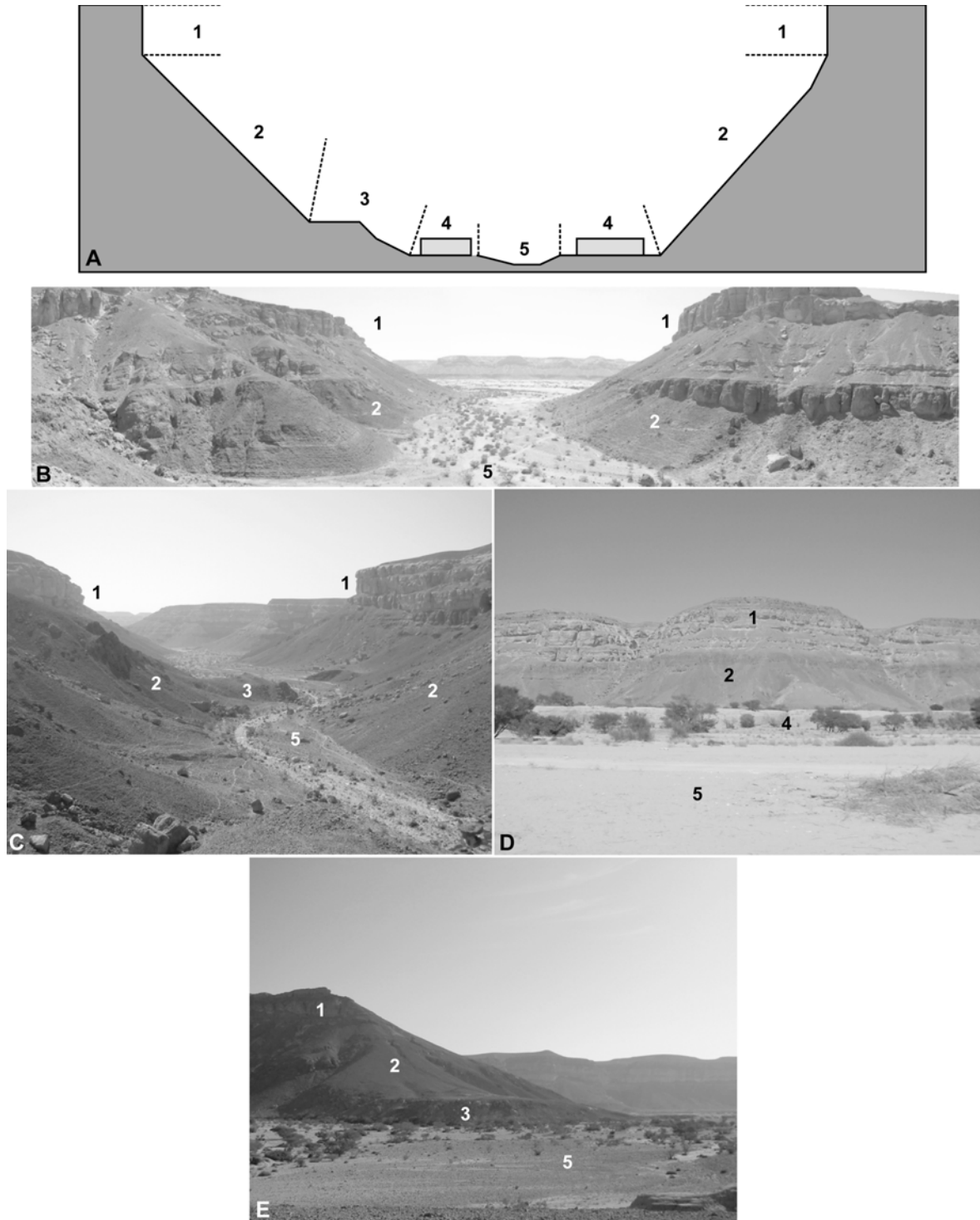
FIGURE 13. A. Coupe schématique de wadi ; B. Wādī Dhhabla ; C. Wādī Jabb ; D-E. Wādī al-Khūn ; Géo-systèmes : 1. falaise et plateau (jawl) ; 2. cône de déjection ; 3. terrasse au pied d'un cône de déjection ; 4. terrasse de limons ; 5. fond de wadi.
