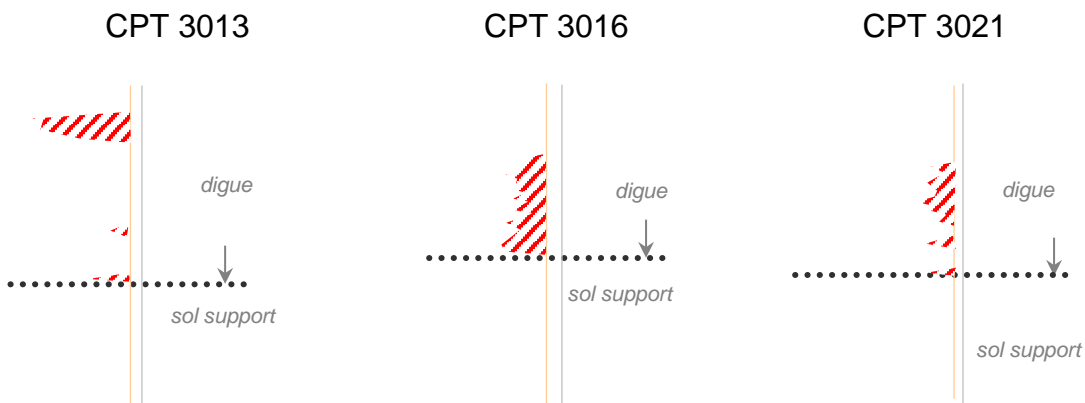
Figure 7. Interprétation des résistances de pointe des sondages CPT3013, 3016 et 3021 exprimées en densité relative en fonction de la profondeur selon Baldi. En hachuré rouge, les zones d'indice de densité inférieur à 40%.
