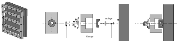
Figure 4 : Description de la conception du châssis à ressort
