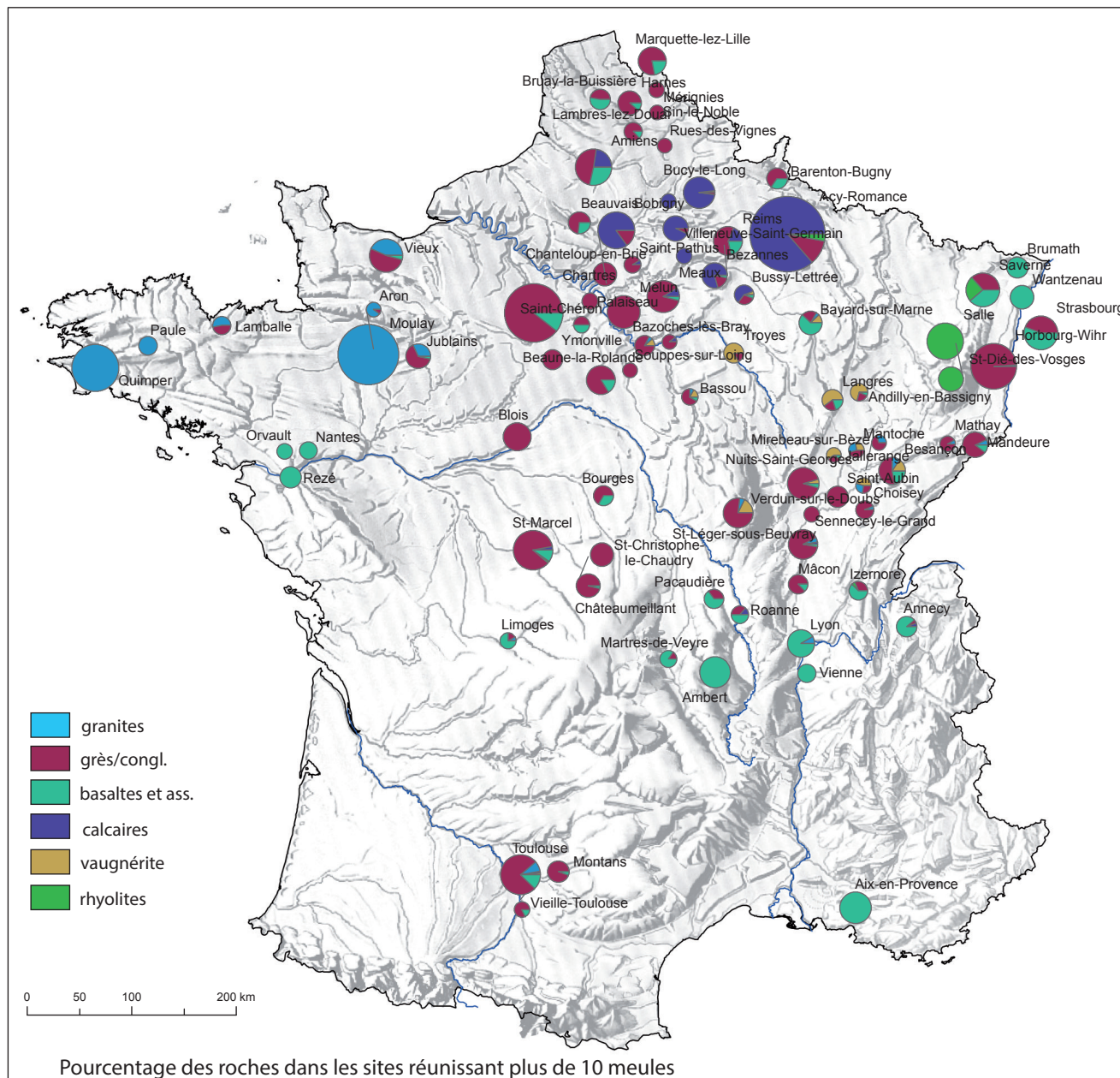
Fig. 1. Principaux matériaux constitutifs (niveaux 1) des meules rotatives (base de données 2014).
