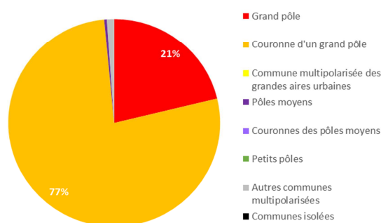
Figure 44 : Durées cumulées comparées des arrêts, selon le ZAU, entre espaces ruraux polarisés et isolés – BF, 2016
