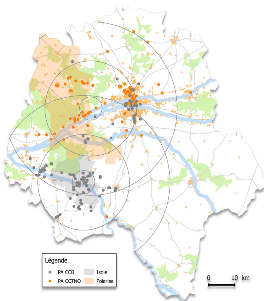
Figure 34 : Illustration du calcul de dispersion, par classe de distance, des points d'arrêt autour de quelques lieux de résidence – BF, 2015
