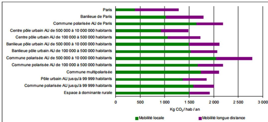
Figure 12 : Emissions annuelles de CO2 liées aux déplacements selon le lieu de résidence, par habitant
