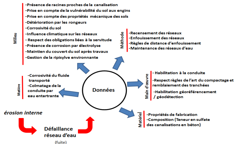
Figure 2. Identification et classification des causes de la défaillance (fuite) d'une canalisation d'eau déclenchant un mécanisme d'érosion interne dans la digue selon la méthode des 5M
