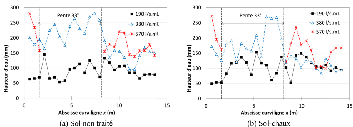
Figure 6 : Hauteurs d'eau mesurées dans l'écoulement en cours d'essai par règle graduée pour le sol non traité (a) et le sol-chaux (b). Le zéro de l'abscisse curviligne se situe en crête.
