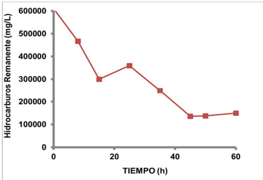
FIGURA 2. Curva de remoción de hidrocarburos totales por BFNA en un agua tratada proveniente de un centro de lavado automotriz.
