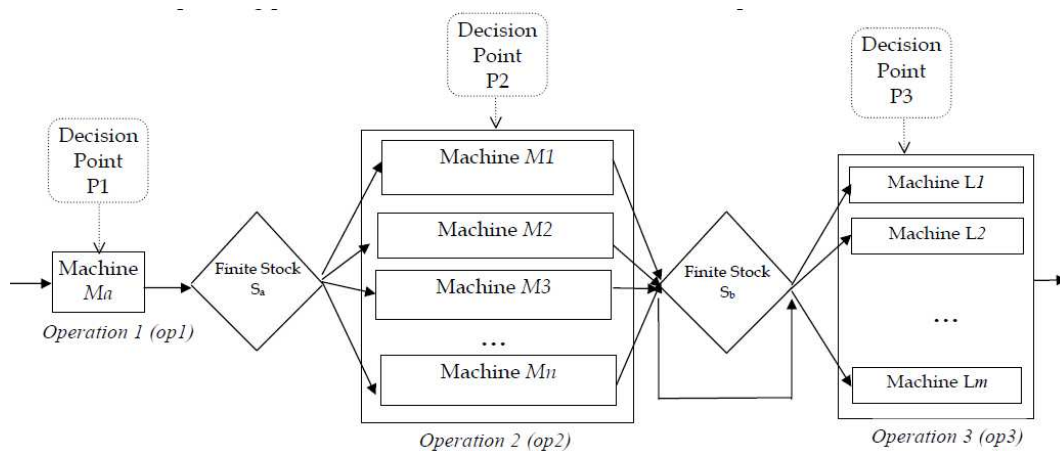
Figure 7. Flowshop hybride à 5 étages
