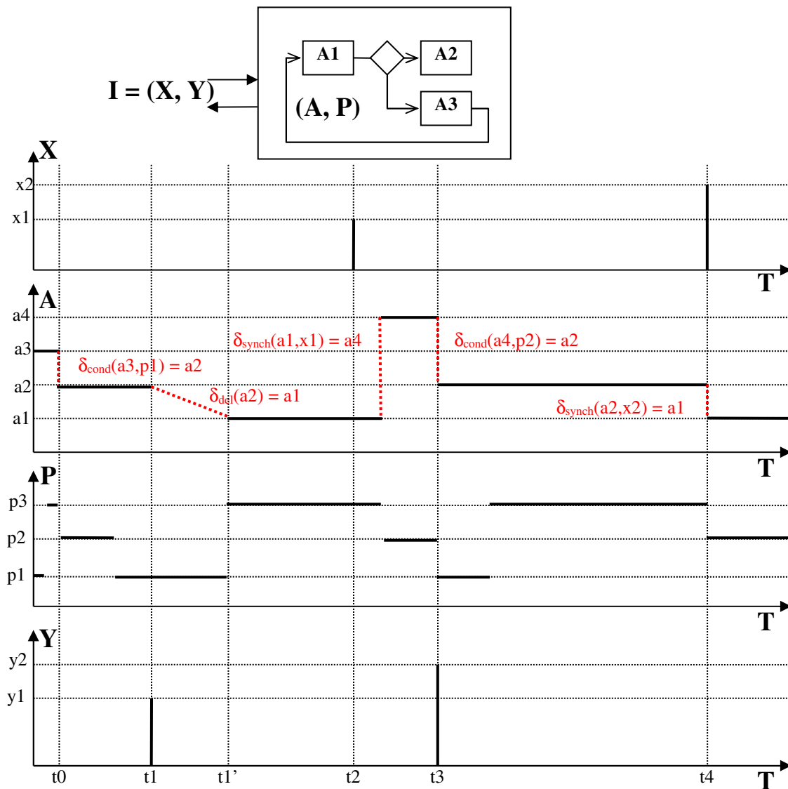
Figure 16. Comportement en MoC AC de système
