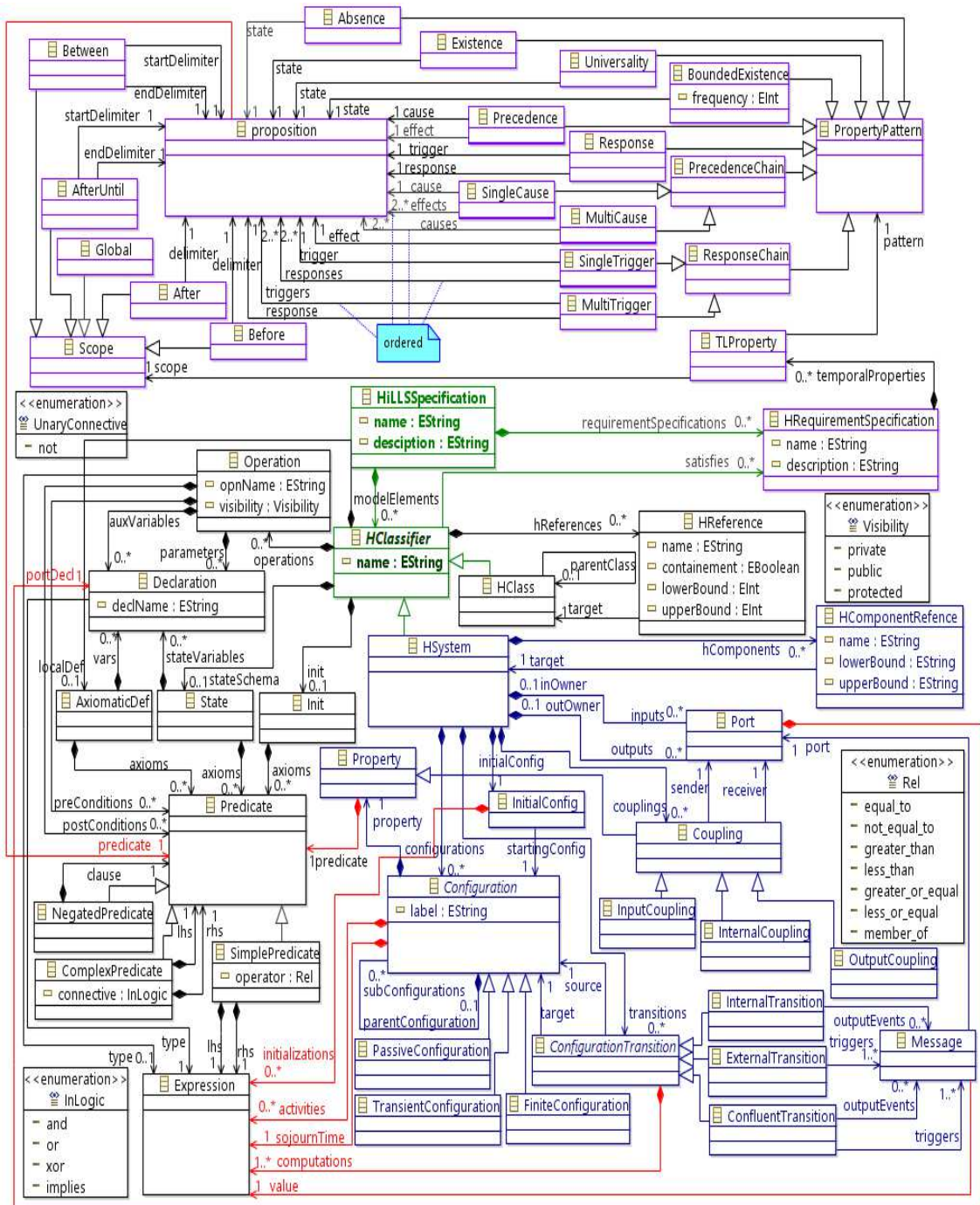
Figure 34. Syntaxe abstraite de HiLLS
