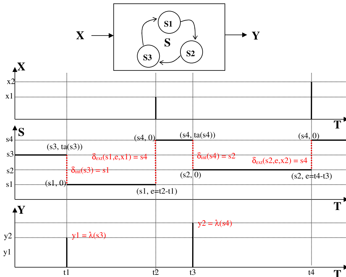
Figure 15. Comportement en MoC EE de système
