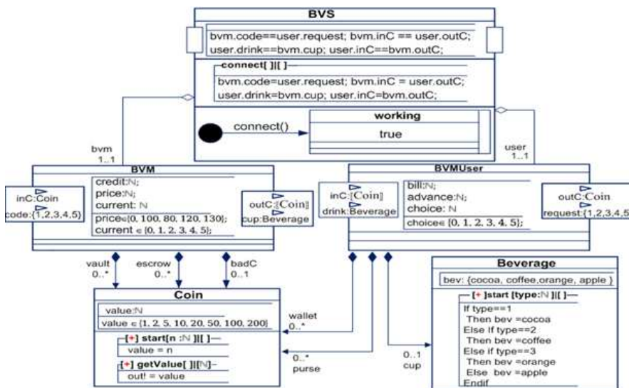
Figure 33. Modèle HiLLS du système de distribution de boisson
