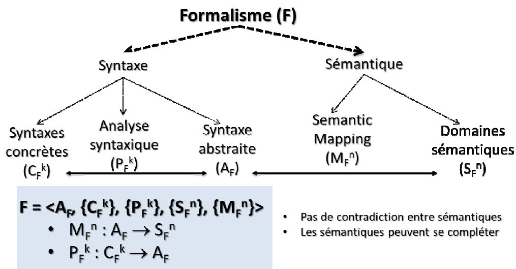
Figure 23. Langage multi-sémantique
