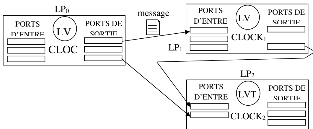
Figure 35. Architecture générique de simulation répartie
