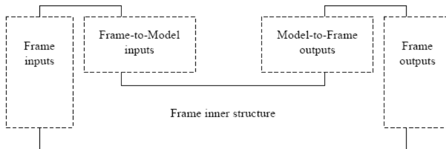
Figure 41. Approche « plug-in »
