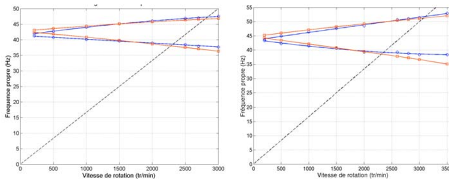
Figure 8. Diagrammes de Campbell expérimentaux (rouge) et numériques (bleu) pour deux configurations (gauche= configuration 2, droite=configuration 3)
