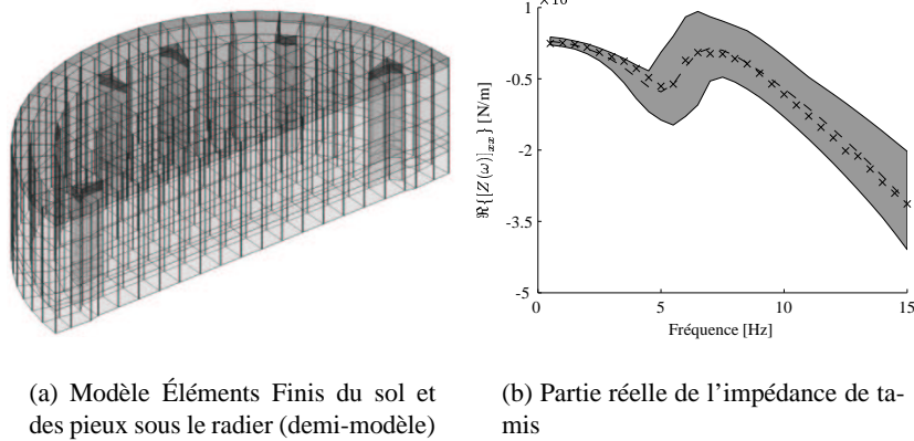
Figure 2. Application de la méthode non paramétrique au calcul de l'impédance de tamis du sol et des pieux d'une cuve de stockage de gaz : résultat déterministe (+), modèle moyen (—) et enveloppe des tirages de Monte-Carlo (en gris).
