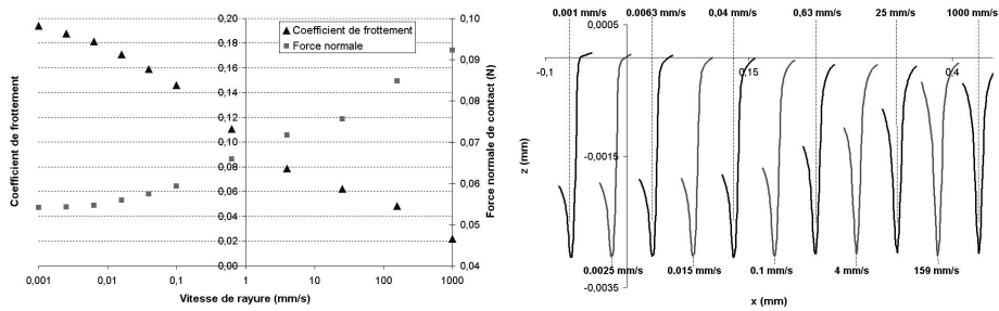
Figure 4. Rayure d'un solide élastique-viscoplastique, A gauche - Effort de contact et coefficient de frottement en fonction de la vitesse de rayure, A droite - Profil longitudinal pour différentes vitesses de rayure
