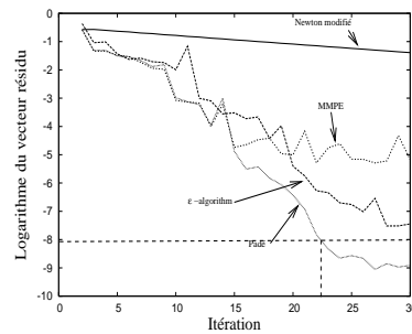
Figure 3. Evolution de la norme du résidu en fonction des itérations de Newton-modifié. Comparaison des trois méthodes d'accélération de la convergence.
