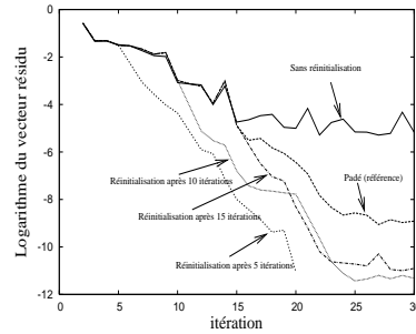
Figure 4. Evolution de la norme du résidu en fonction des itérations de Newton-modifié. Trois essais de réinitialisation du MMPE : après 5, 10 et 15 itérations.
