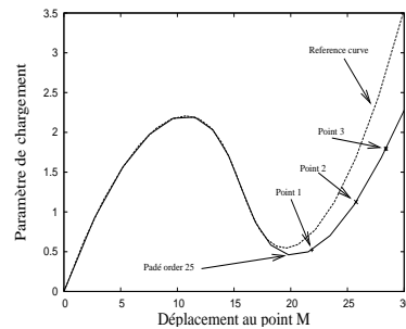
Figure 2. Visualisation des points à corriger sur la courbe de réponse.
