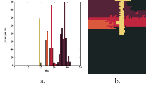
FIGURE 3. Résultat de la segmentation d'histogramme [9]. (a) l'histogramme segmenté (bins de 50cm), (b) le résultat dans la carte de profondeur avec les mêmes couleurs.
