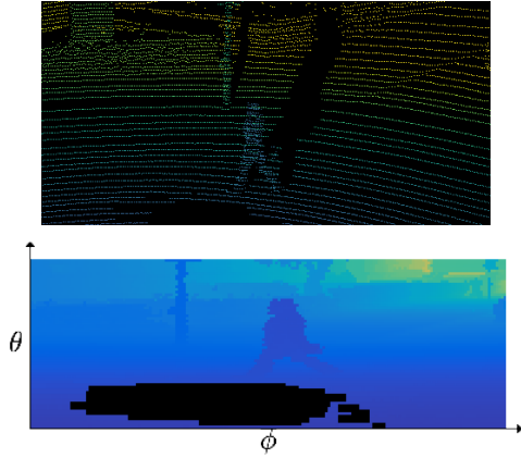
FIGURE 2. Exemple de nuage de points du jeu de données KITTI [11] (haut) transformé en carte de profondeur (bas). Les zones sombres correspondent à des pulsions sans retours du capteur LIDAR.
