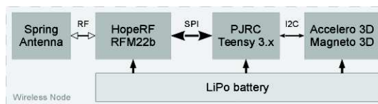
Figure 11. Architecture du nœud WiNo spécifique au projet CANetÁ
