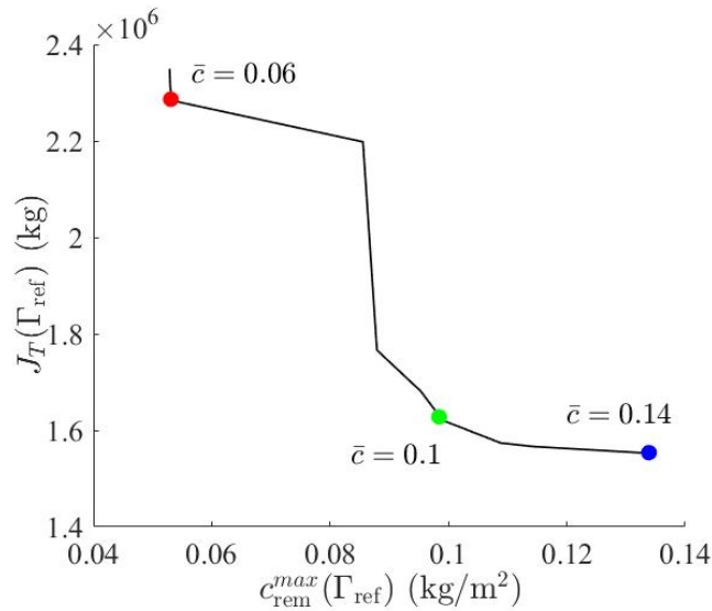
(b) Objective values J_T(\Gamma_{\text{ref}}^{\text{opt}}), c_{\text{rem}}^{\text{max}}(\Gamma_{\text{ref}}^{\text{opt}}) associated to the optimal refilling locations in (a). The black curve represents the Pareto Front. (b) Valeurs des objectifs J_T(\Gamma_{\text{ref}}^{\text{opt}}), c_{\text{rem}}^{\text{max}}(\Gamma_{\text{ref}}^{\text{opt}}) associées aux emplacements optimaux de recharge en (a). La courbe noire représente le Front de Pareto.
