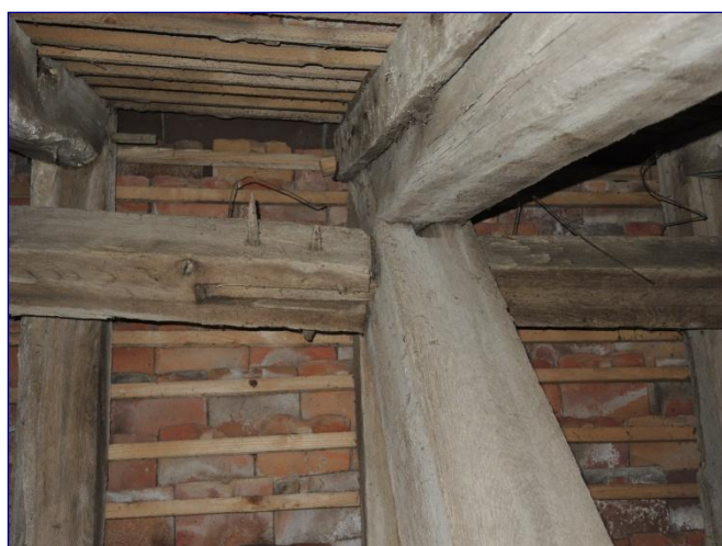
Charpente de la nef, assemblage faîtière et poinçon
