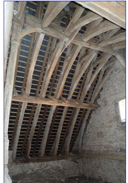
Charpente du chœur, côté nord
