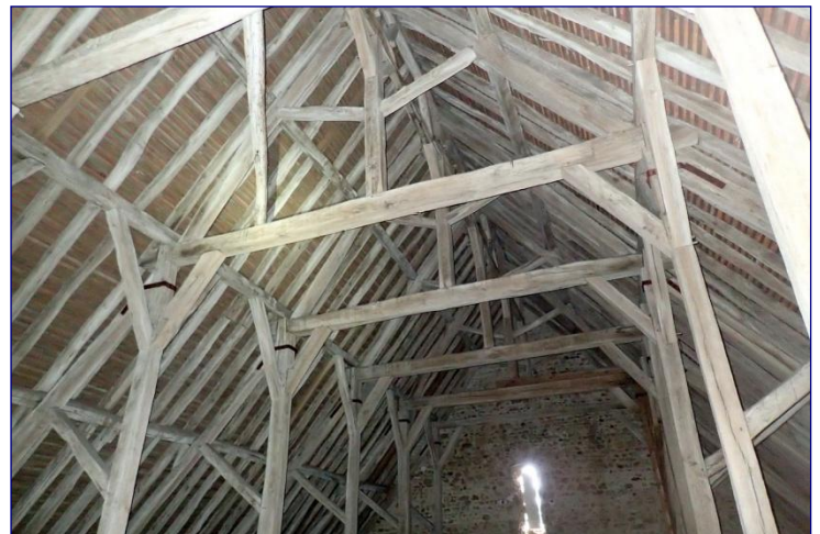
Fig. 12 : partie occidentale de la charpente vers l'ouest
