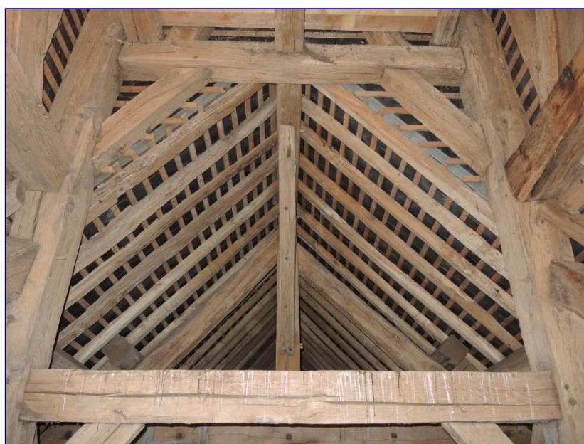
Fig. 16 : charpente de la nef, base du clocher de charpente (paroi est, face ouest)
