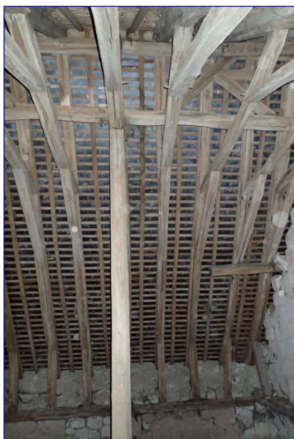
Charpente de la nef, contreventement
