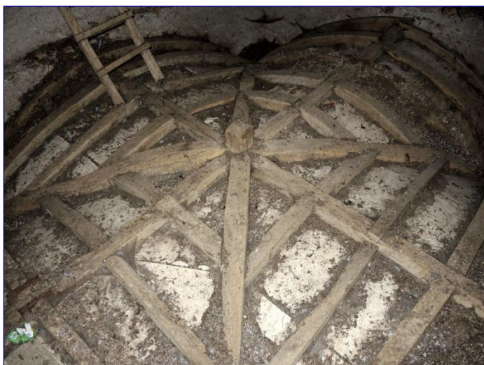
Voûte suspendue de la chapelle nord
