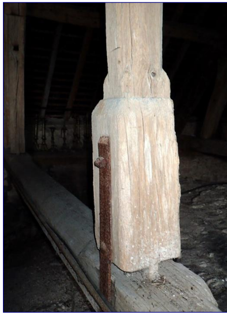
Charpente du vaisseau, pied de poinçon
