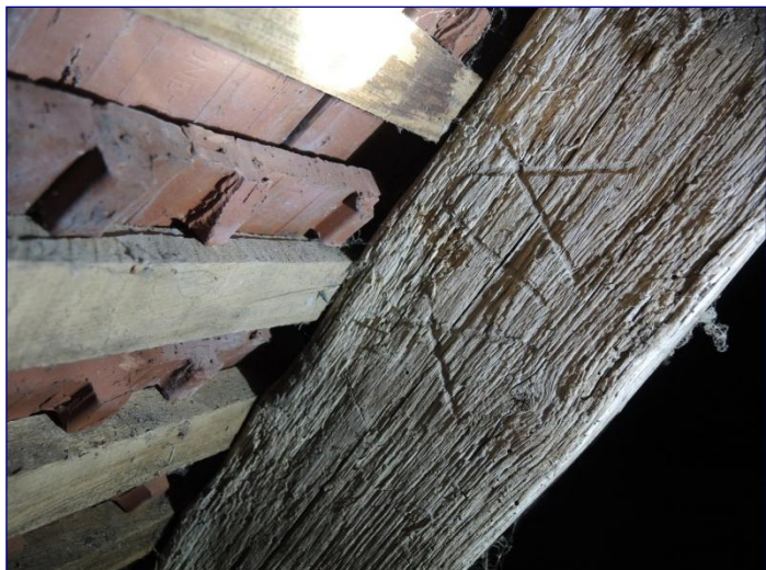
Fig. 11 : charpente est du chœur, marque XIX sur F19
