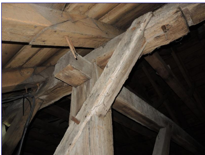
Fig. 10 : charpente de la nef, pan-de-bois longitudinal nord, poteau n° 8, assemblage de la traverse par enfourement
