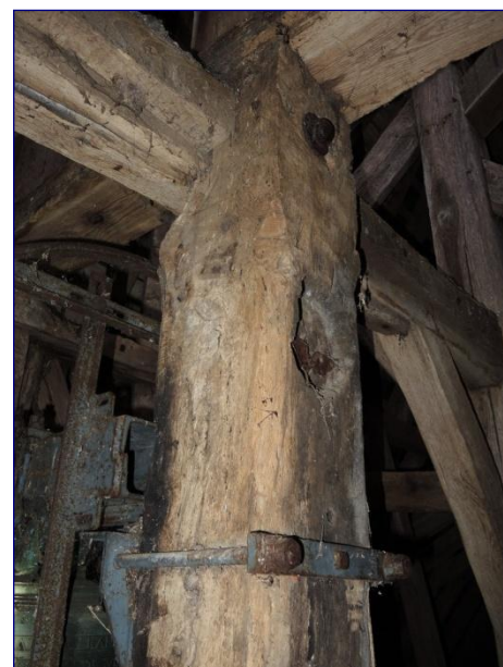
Poinçon bas de la flèche du chœur
