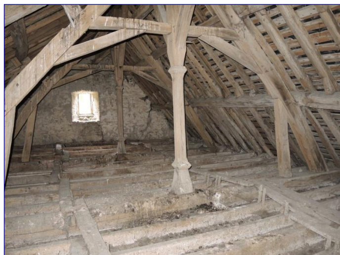
Charpente de la nef vers l'ouest
