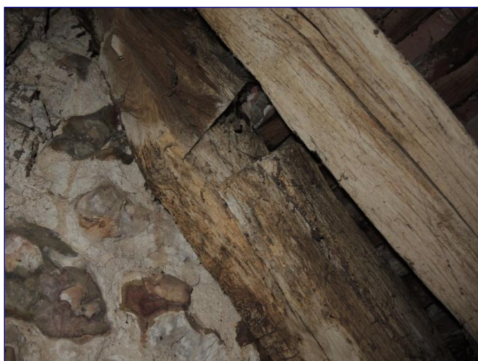
Charpente du chœur, travée est, chevron en remploi
