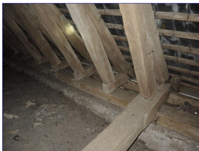
Charpente de la nef, pied des chevrons renforcés par des jambettes
