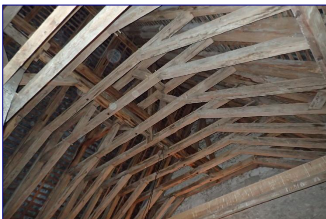
Charpente du chœur, vue générale vers l'ouest
