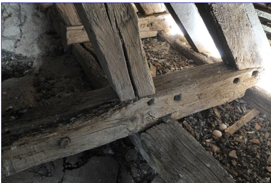
Fig. 12 : charpente de la nef, 1 er entrant au nord avec trous de levage
