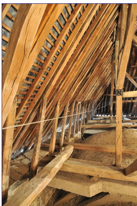
Fig. 10 : charpente du chœur, croupe
