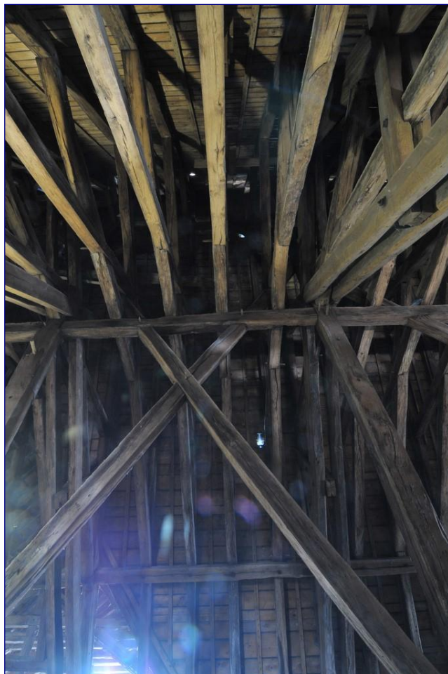
Fig. 5 : charpente de la nef, écharpes croisées entre poinçons
