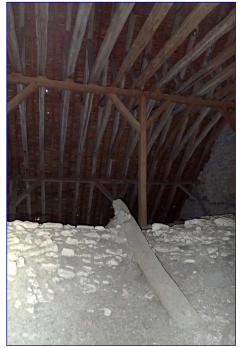
Fig. 5 : partie orientale de la charpente, vestiges d'écharpes croisées
