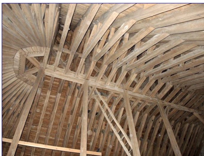
Charpente du chœur, parties hautes
