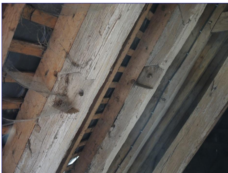
Fig. 7 : chevrons en remplis
