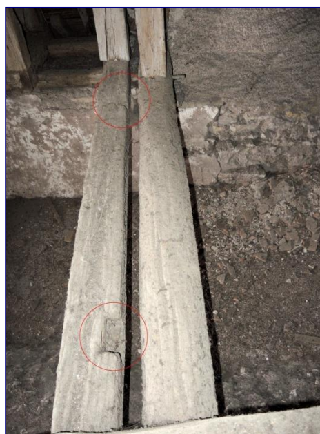
Fig. 12 : charpente de la nef, structure ouest, entailles sur ancien entrait (après 1107d)
