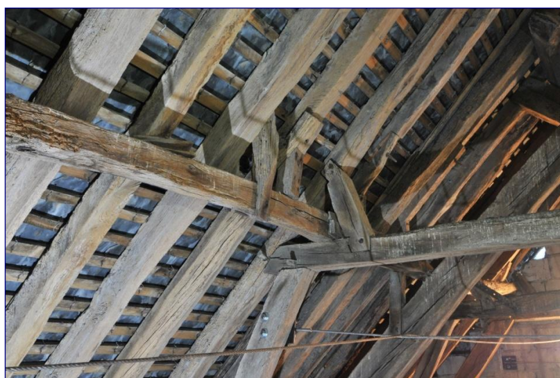
Fig. 9 : charpente du chœur, blocage d'une panne au sud
