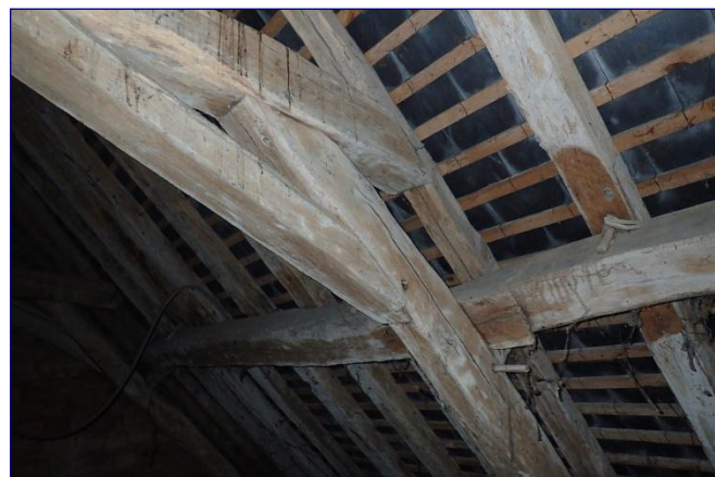
Charpente du chœur, détail d'une ferme
