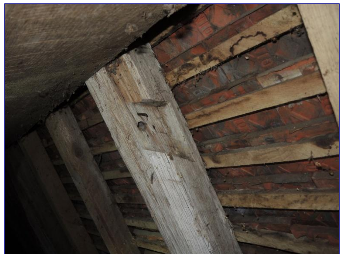
Charpente du chœur, travée ouest, chevron avec mi-bois (pièce en remploi)
