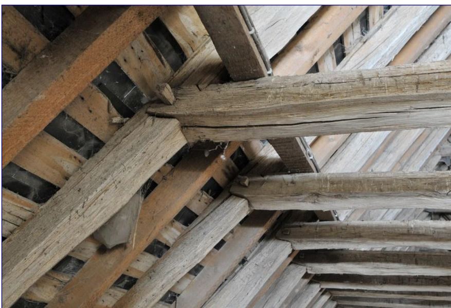
Fig. 9 : charpente de la nef, assemblage des faux-entraits aux chevrons
