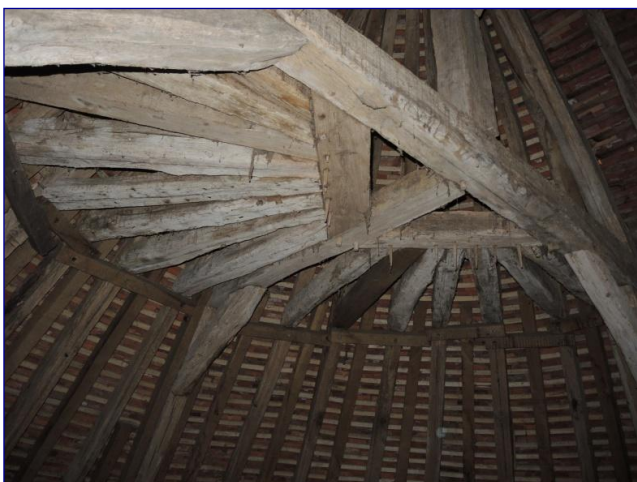
Fig. 7 : charpente du chœur, enrayure haute de l'abside
