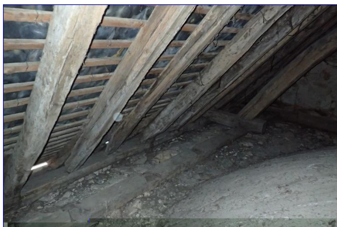
Charpente du chœur, pieds de ferme
