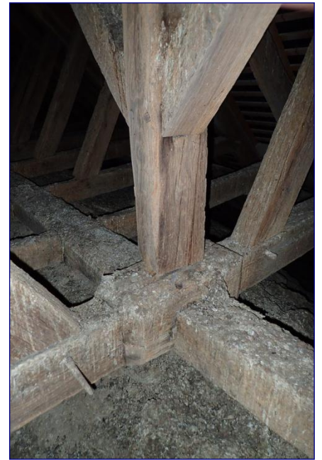
Structure orientale, pied du poinçon haut
