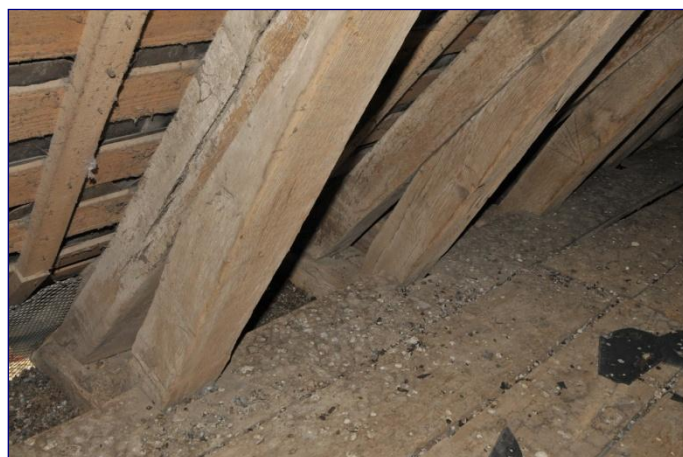
Charpente de la nef, détail des pieds de ferme
