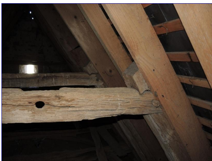
Fig. 8 : charpente du chœur, assemblage à mi-bois
