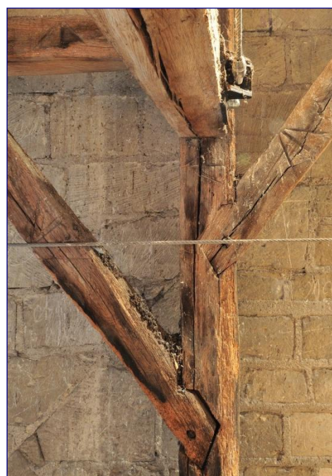
Fig. 11 : charpente du chœur, assemblages à mi-bois
