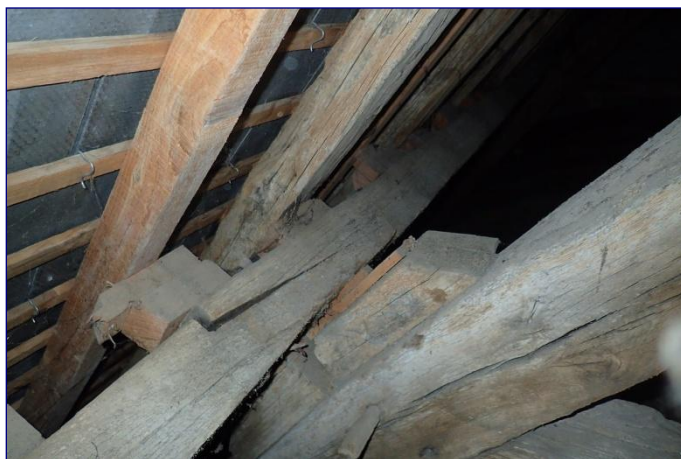
Charpente de la nef, assemblage par enture des pannes
