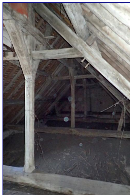
Charpente de la nef vers l'ouest
