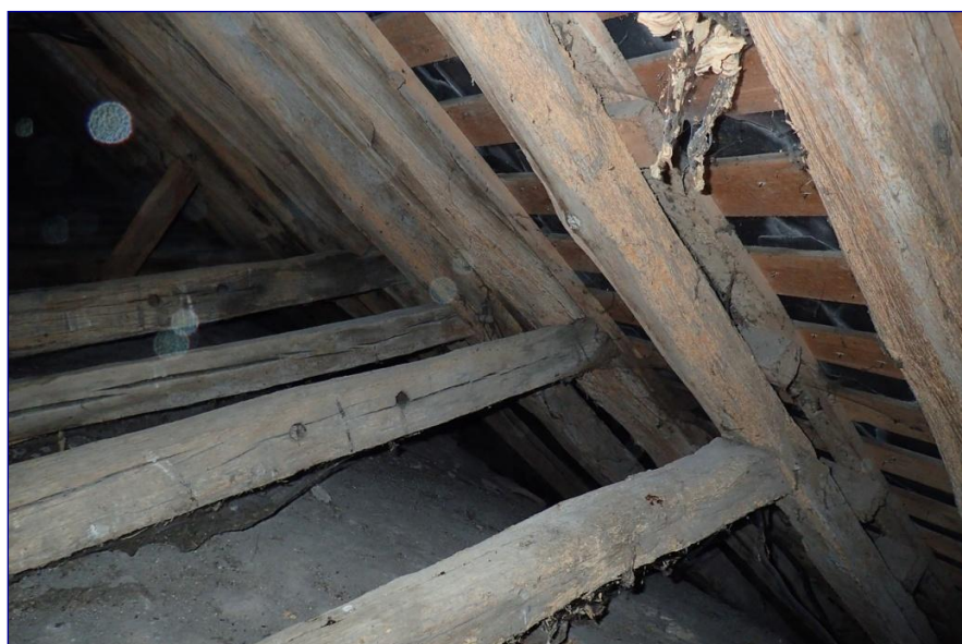
Fig. 9 : charpente du chœur, assemblages des entrails retroussés avec les chevrons (F6 et F8 à mi-bois)
