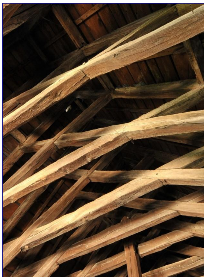
Fig. 9 : charpente du bras nord, assemblage à mi-bois des écharpes
