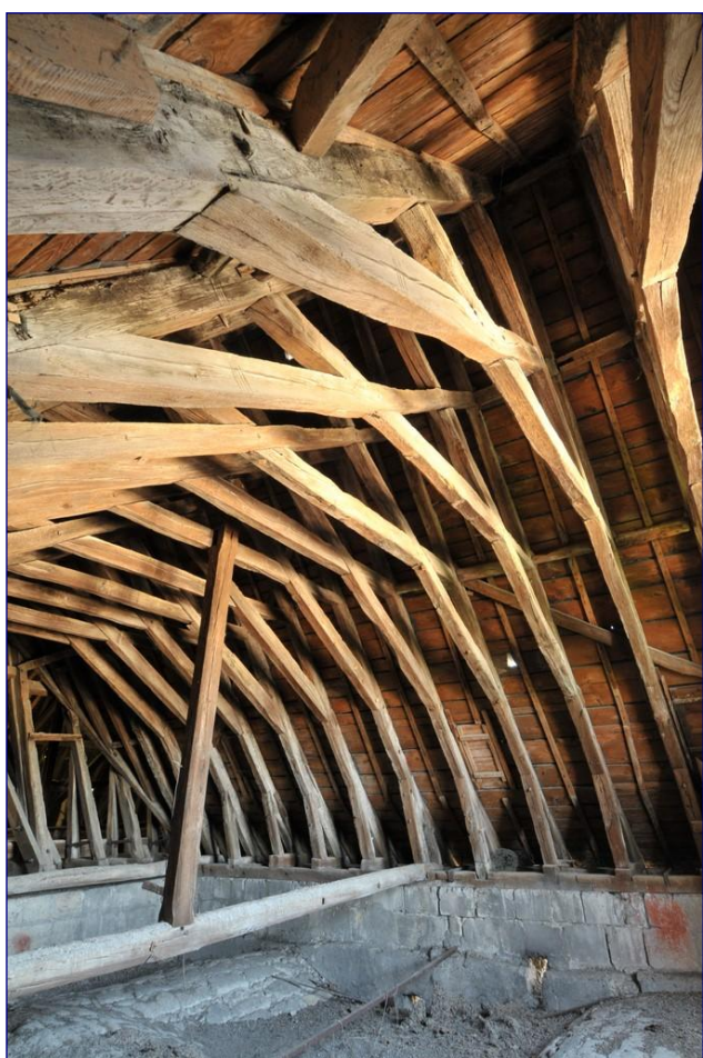
Fig. 8 : charpente du bras nord, vue générale vers l'ouest
