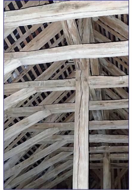
Charpente de la nef, poinçon d'une ferme
