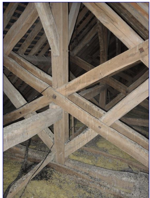
Charpente de la nef renforcée par des moises
