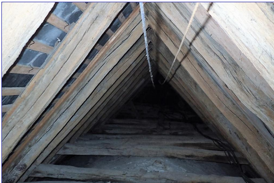
Fig. 8 : charpente du chœur, chevrons-formant-ferme reliés par un entrait retroussé
