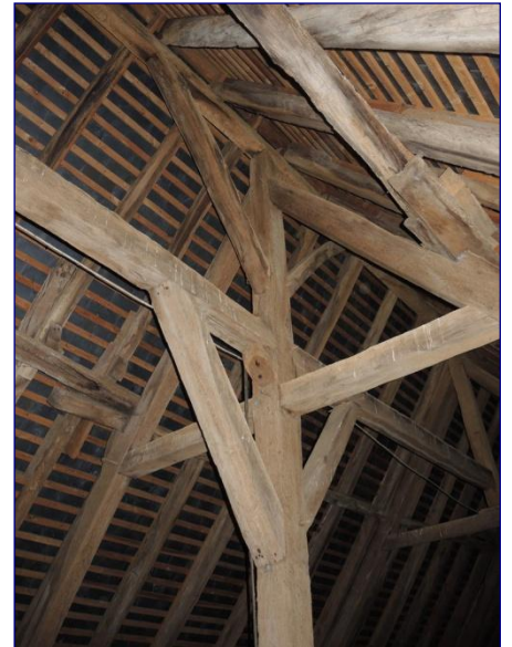
Charpente de la nef, détail d'un poinçon
