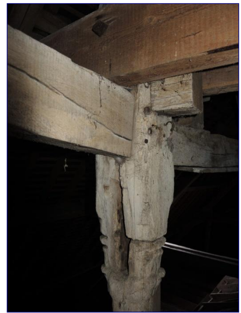
Charpente de la nef, poinçon sculpté de F2
