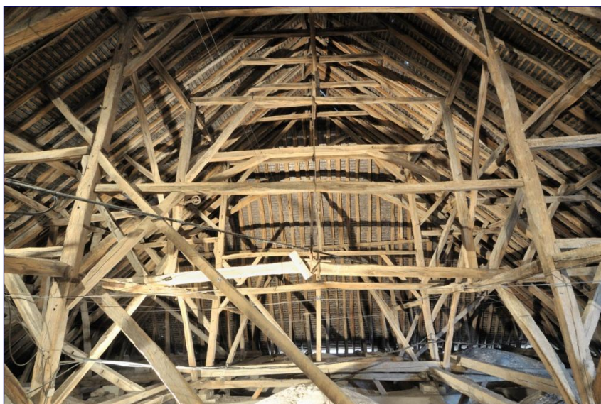
Fig. 7 : charpente du chœur
