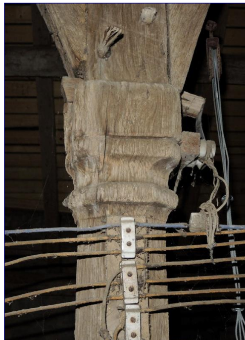
Fig. 10 : charpente de l'avant-chœur, chapiteau de poinçon
