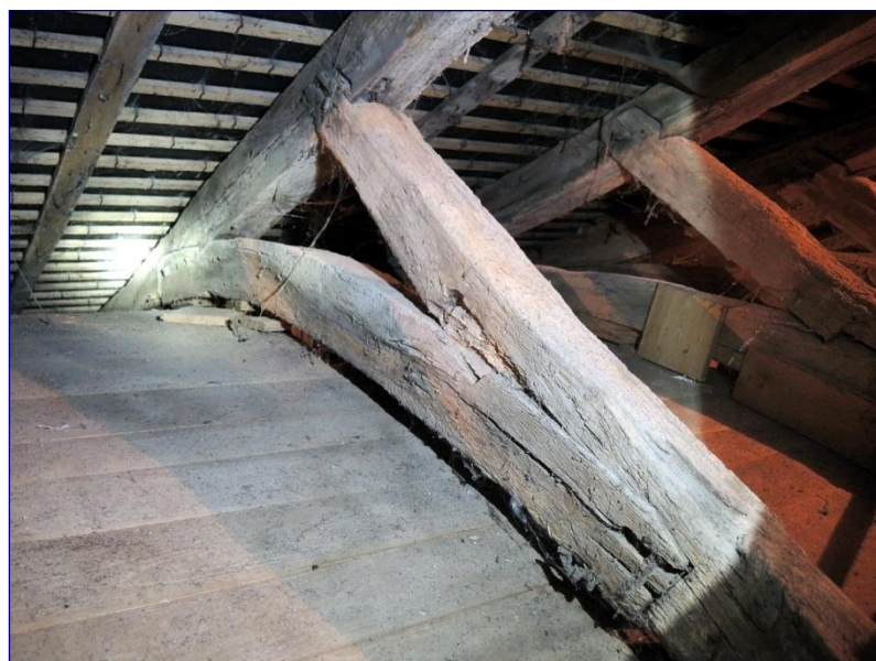
Fig. 9 : charpente de la nef, un faux-entrait et son aisselier
