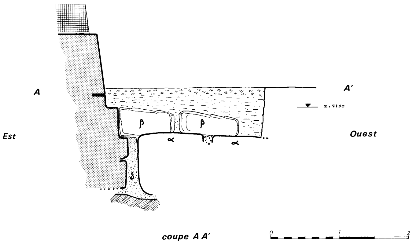
2. Coupe du sondage. (Relevé et dessin L. Gabolde).
