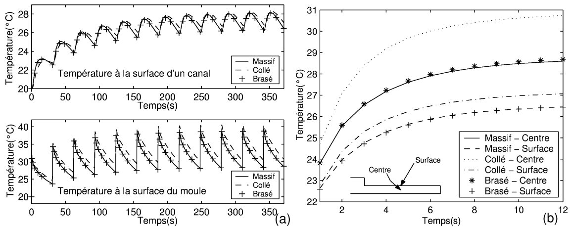
FIG. 5 – Effet de la stratification sur la température du moule (a) et de la pièce en fin de cycle (b)
