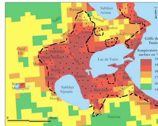
Figure 9. Champ thermique de surface nocturne dans l'agglomération de Tunis par temps radiatif à partir d'une scène NOAA-AVHRR datée du 04/06/2001 à 1h26 TU. En pointillés : limites de la forte urbanisation. D'après Charfi, 2012 modifié.
