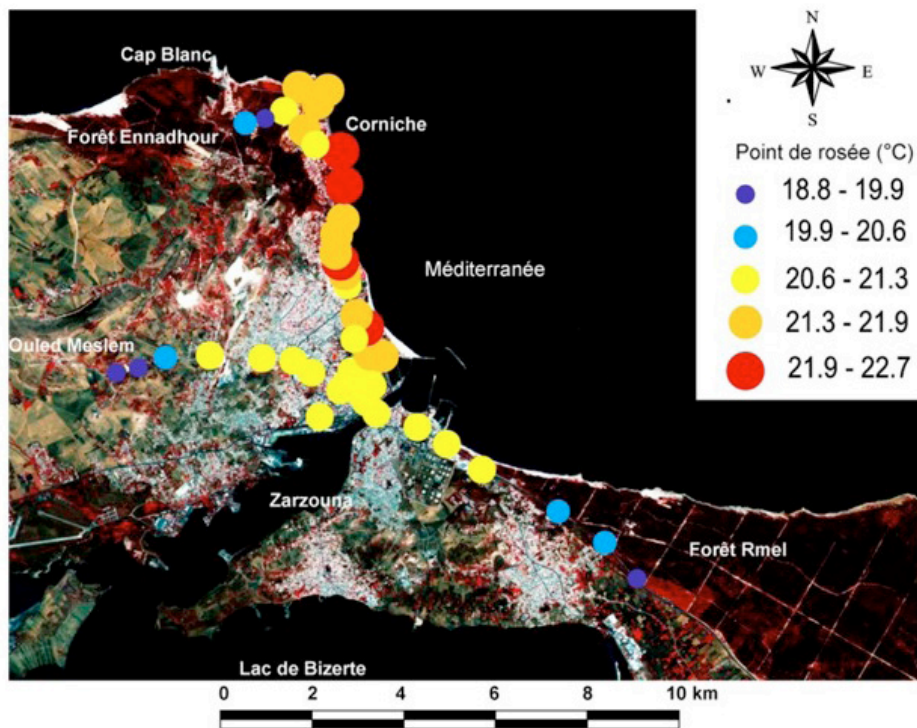
Figure 6 : Variation spatiale de la température de rosée nocturne dans l'agglomération de Bizerte (mesures itinérantes par temps radiatif le 5 août 2016 ; fond, composition colorée fausses couleur infrarouge d'une scène Landsat 8 datée du 4 août 2016).
