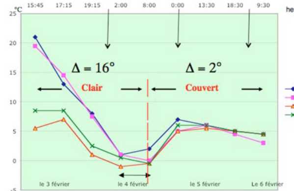
Figure 4. Températures de la surface des murs extérieurs d'une maison selon leur orientation et la nébulosité, du 3 au 6 février 2005 près de Nice.
