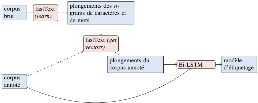
(b) fastText
