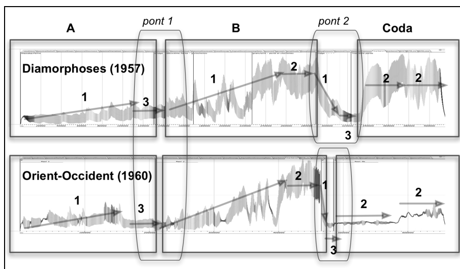
Figure 25. Comparaison des articulations formelles. (L'original est en couleur)
