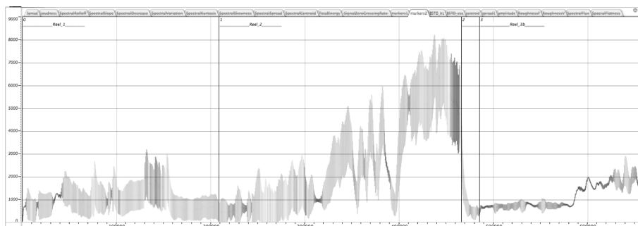
Figure 20. Alignement de la représentation avec la segmentation proposée par Solomos [Solomos 2009a]. (L'original est en couleur)
