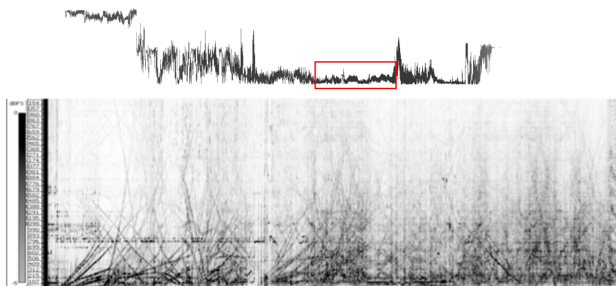
Figure 6. Spirals in La Légende d'Eer (24'50'' – 33' 08'').
