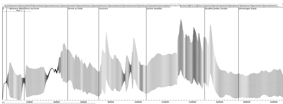
Figure 17. Première section d' Orient-Occident et les évènements du film. (L'original est en couleur)
