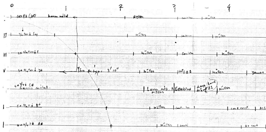
Figure 2. The beginning of La Légende d'Eer .
