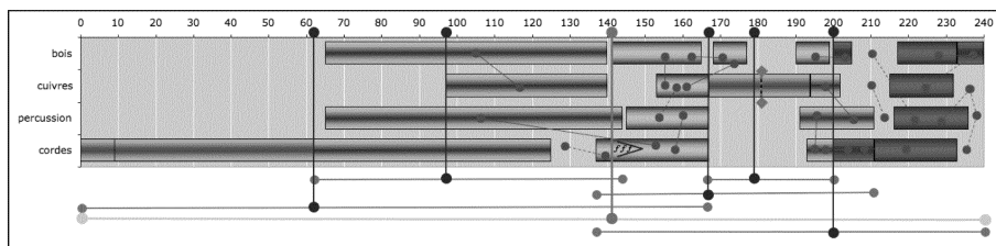
Fig. 2. Jonchaies : organisation structurelle des parties de la structure ainsi que de la disposition des groupes instrumentaux. Proportions d'or marquées par les lignes horizontales. [L'original est en couleur]
