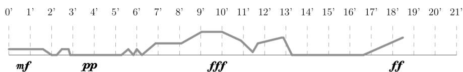
Ex. 3. Bohor , profil dynamique de la voie Orgue.
