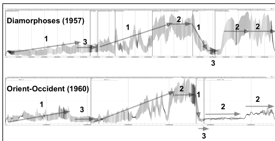
Figure 24. Superposition des représentations et catégories. (L'original est en couleur)
