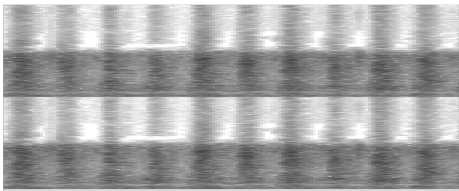
Figure 2. Spectrogramme du fichier audio compressé 4 .
