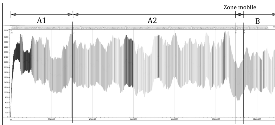
Figure 27. Résumé analytique selon Couprie [Couprie 2007], par rapport à l'évolution de la masse sonore. (L'original est en couleur)
