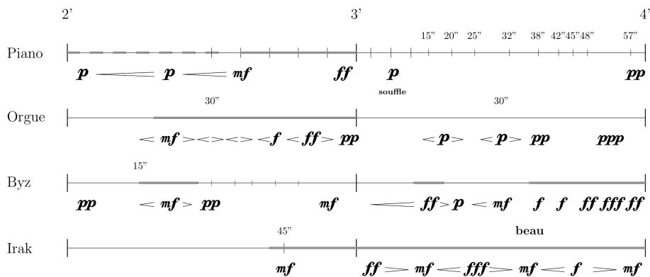
Ex. 7. Bohor , 2'-4': plan graphique.
