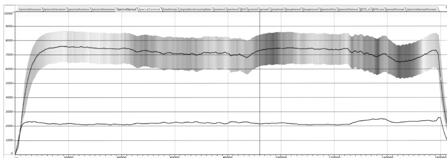
Figure 10. L'évolution de la « masse sonore » et de la variance spectrale de Concret PH (1958). (L'original est en couleur)
