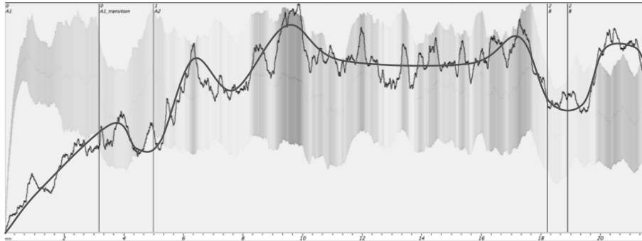
Figure 30. Lissage de la courbe d'évolution de l'énergie. (L'original est en couleur)
