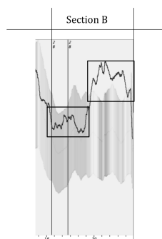
Figure 33. Articulation de la section « B » de Bohor , par l'accroissement d'énergie. (L'original est en couleur)
