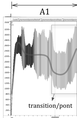
Figure 28. Le pont entre les sections A1 et A2. (L'original est en couleur)
