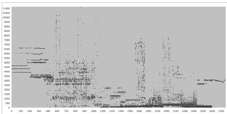
Fig. 8. La Légende d'Eer. Représentation graphique de l'analyse des 30 premiers composants spectraux du son.
