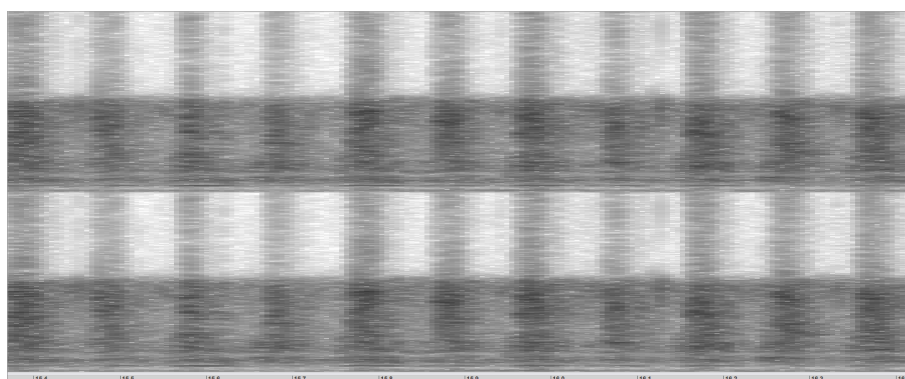
Figure 1. Spectrogramme du fichier original 3 .
