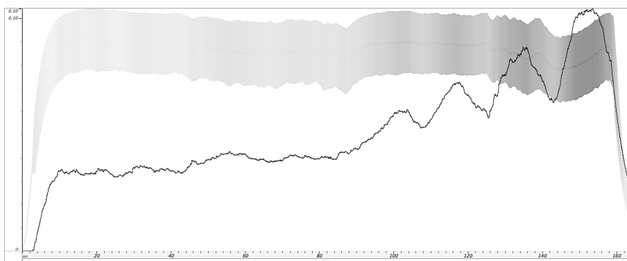
Figure 14. Evolution de la « planéité spectrale » de Concret PH (1958). (L'original est en couleur)
