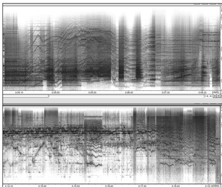
Fig. 11. Début de la deuxième section de Jonchaies (en haut) et de La Légende d'Eer (en bas).
