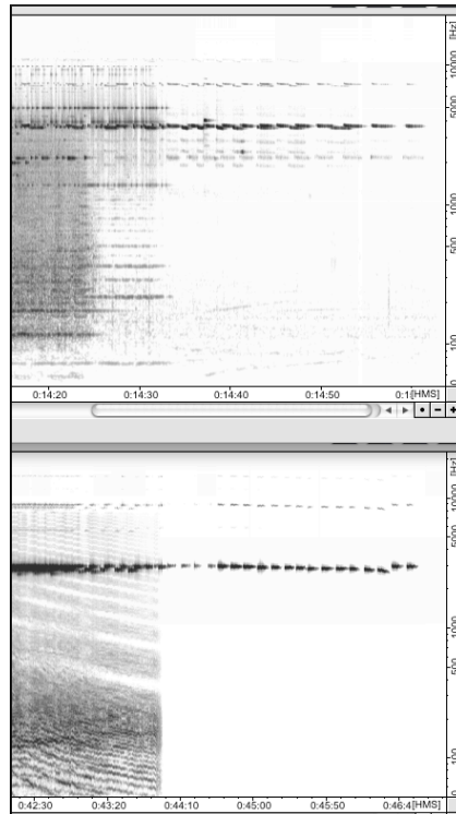
Fig. 13. Détail de la fin de Jonchaies (en haut) et de La Légende d'Eer (en bas).
