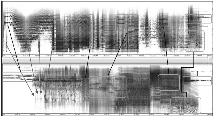
Fig. 14. Similitudes entre Jonchaies (en haut) et La Légende d'Eer (en bas) visibles dans les spectrogrammes des œuvres.
