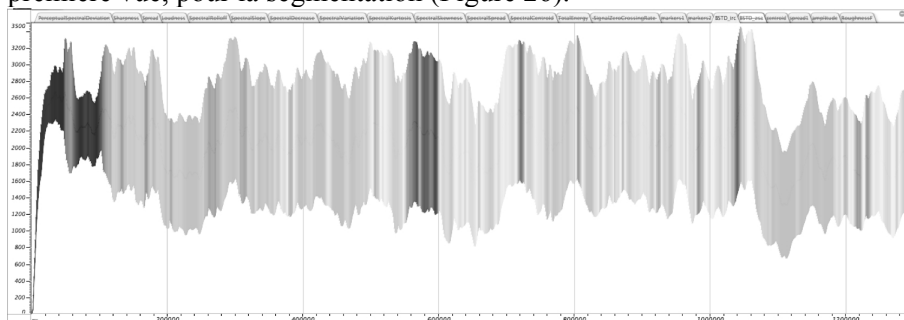
Figure 26. Evolution de la “masse sonore” dans Bohor (1962). (L’original est en couleur)
