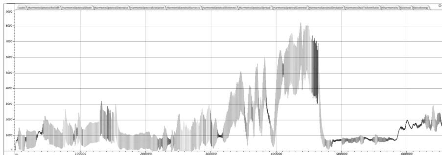
Figure 15. Construction de la représentation d'évolution de la « masse sonore » à partir de la BStD. (L'original est en couleur)
