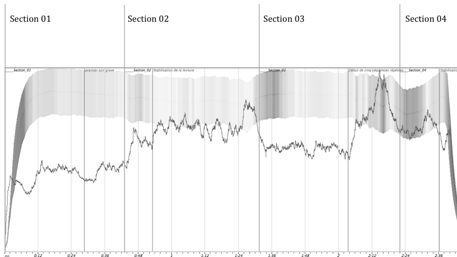
Figure 12. Segmentation à partir de l'évolution de la variation spectrale perceptive de Concret PH (1958). (L'original est en couleur)
