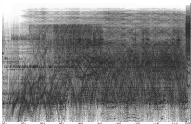
Fig. 5. Section 4 de La Légende d'Eer .
