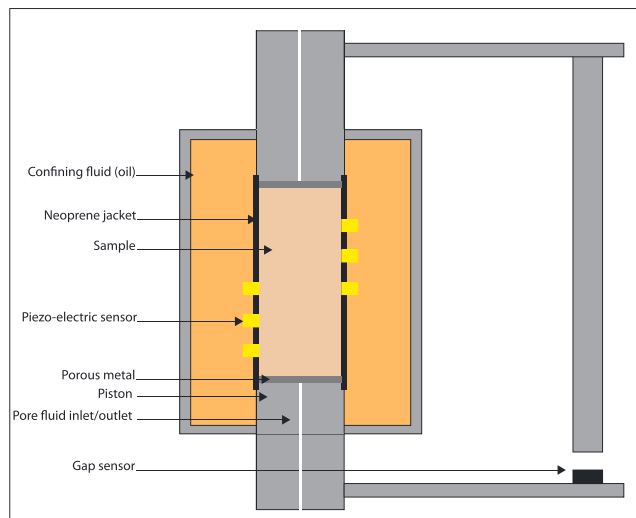
Figure 3. Schematics of the triaxial apparatus at Laboratoire de Géologie of ENS Paris.
