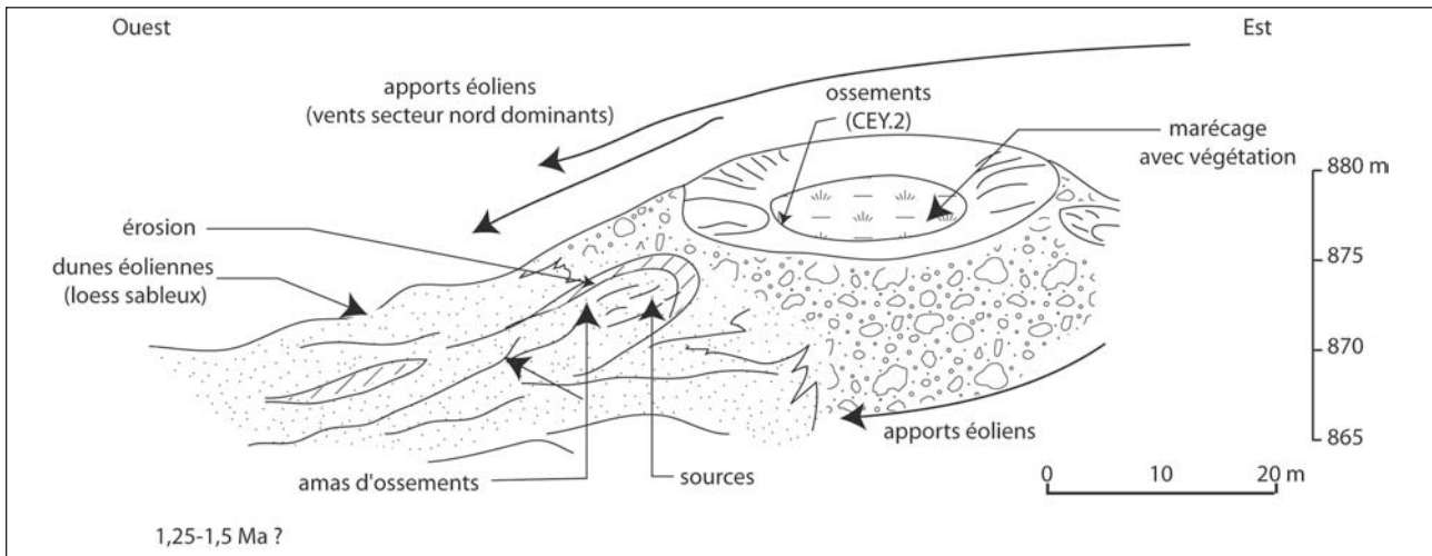
Fig. 1 : Ceysseguet (Haute-Loire). Situation du gisement fossilifère au moment de sa formation sur les pentes du volcan.
