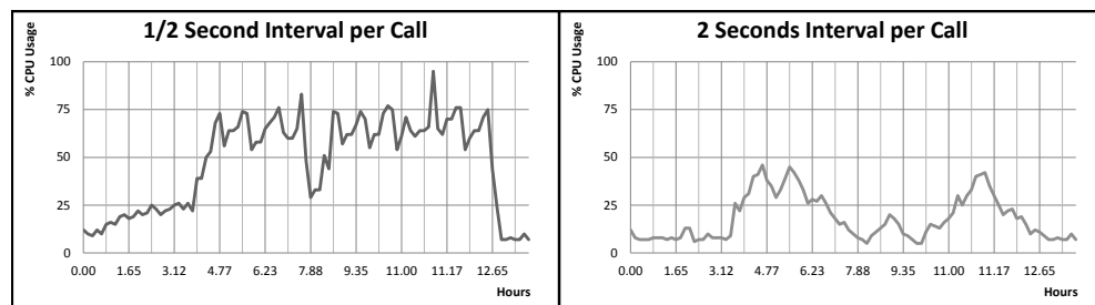
Fig. 4: CPU Usage (1)
