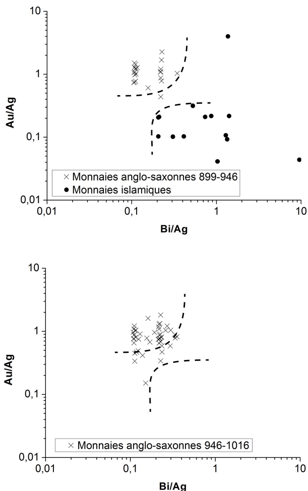
FIGURE 7.6 – Graphiques des rapports Au/Ag en fonction des rapports Bi/Ag, pour les monnaies anglo-saxonnes émises entre 899 et 1016 et pour les monnaies islamiques (d'après [21]).
