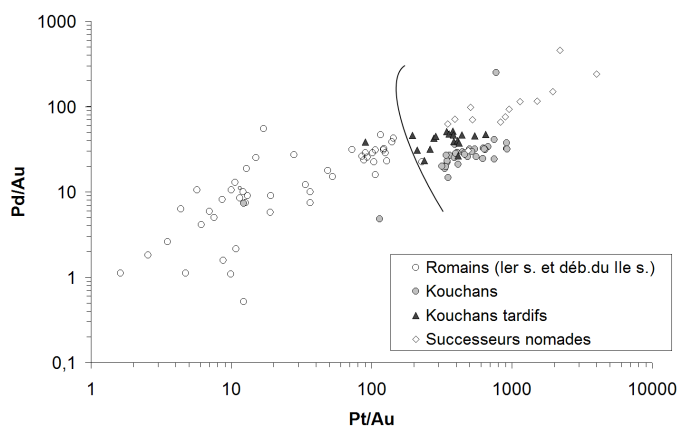
FIGURE 7.4 – Comparaison des rapports Pd/Au et de Pt/Au entre les monnaies d'or kouchanes et romaines (d'après [93]).
