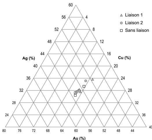
FIGURE 7.7 – Composition des statères au nom de Vercingétorix avec ou sans liaison de coin (d'après [72]).
