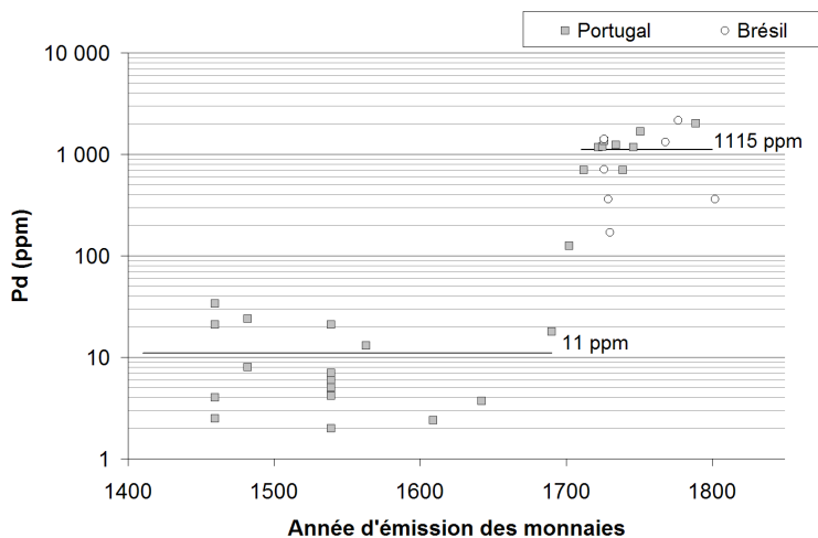
FIGURE 7.3 – Évolution de la teneur en Pd de monnaies d'or portugaises émises entre 1450 et 1800 (d'après [64]).
