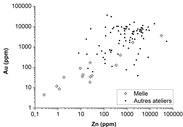
FIGURE 7.2 – Graphique des teneurs en Au en fonction de celles en Zn pour les monnaies en argent de Melle et celles des autres ateliers carolingiens (d'après [75]).
