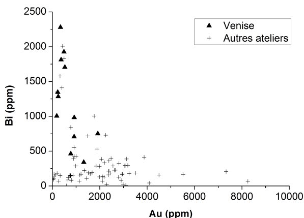
FIGURE 7.5 – Graphique des teneurs en Bi en fonction de celles en Au pour les monnaies en argent de Venise et celles des ateliers carolingiens (d'après [96]).
