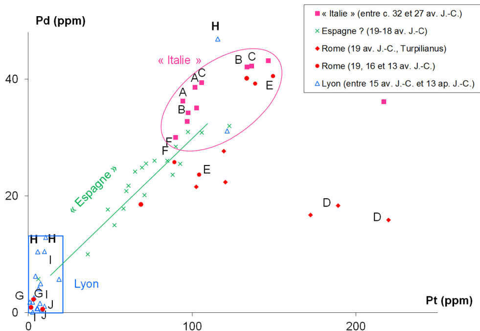
FIGURE 7.10 – Graphique des teneurs en Pd en fonction de celles en Pt pour les monnaies d'or d'Auguste frappées entre 32 av. J.-C. et 4 après J.-C. (d'après [85]). Les monnaies appartenant à un même type sont repérées par une lettre (A à J).
