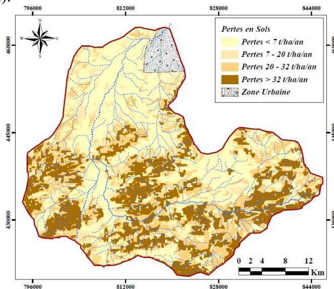
Figure 8 : Carte des pertes en sols dans le Bassin de l’oued Isly
