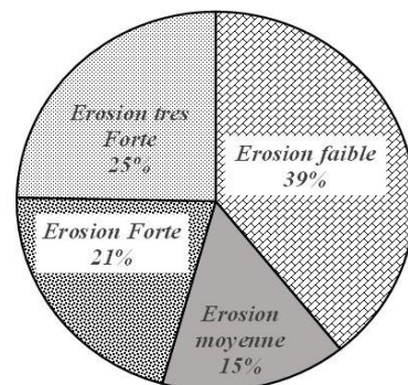
Figure 9 : Répartition des classes d’érosion dans le bassin de l’oued Isly
