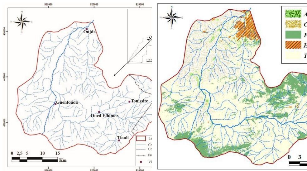
Figure 1 : Bassin versant de l’oued Isly
