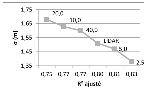
Figure 4 : Comparaison des écarts-types des modèles de H_0 par source de donnée (drone et LiDAR) en fonction du R 2 ajusté.
