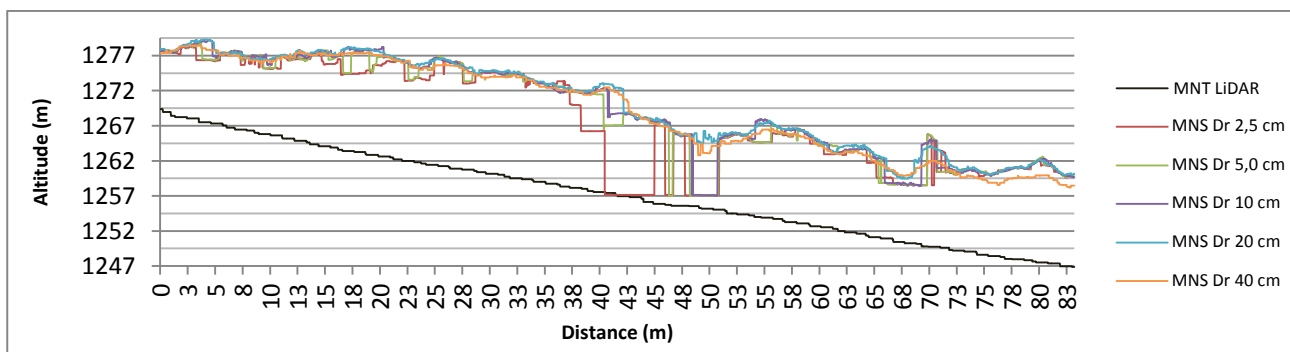
Figure 2 : Profils de points dans la zone SP3 (h) et SP2 (b) avec les MNS du drone aux différentes RS et le MNT LiDAR
