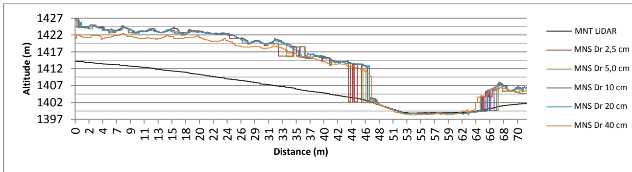
Figure 1 : Zone d'étude SP3 survolée par le drone et mesurée sur une placette d'analyse de 15 m de rayon, MNS calculé à partir des images à 2,5 cm de résolution (a). Le plan de vol avec des recouvrements de 80 % ; les deux bandes de 10 photos ne sont pas prises en lacet mais dans le sens du vent de manière à augmenter l'autonomie du drone (b)
